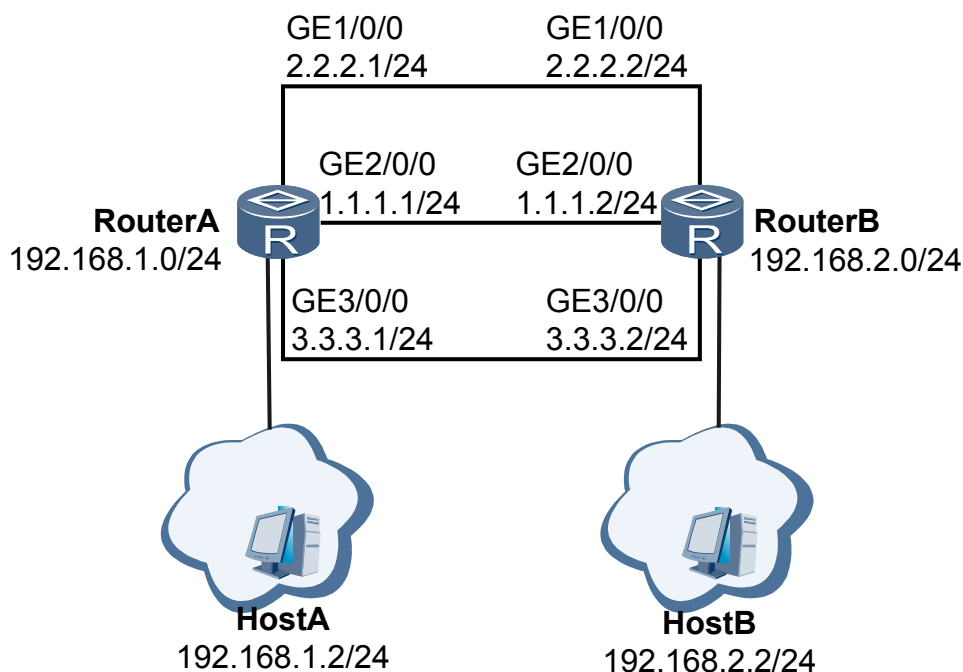
图 1-7 配置主备接口备份组网图
