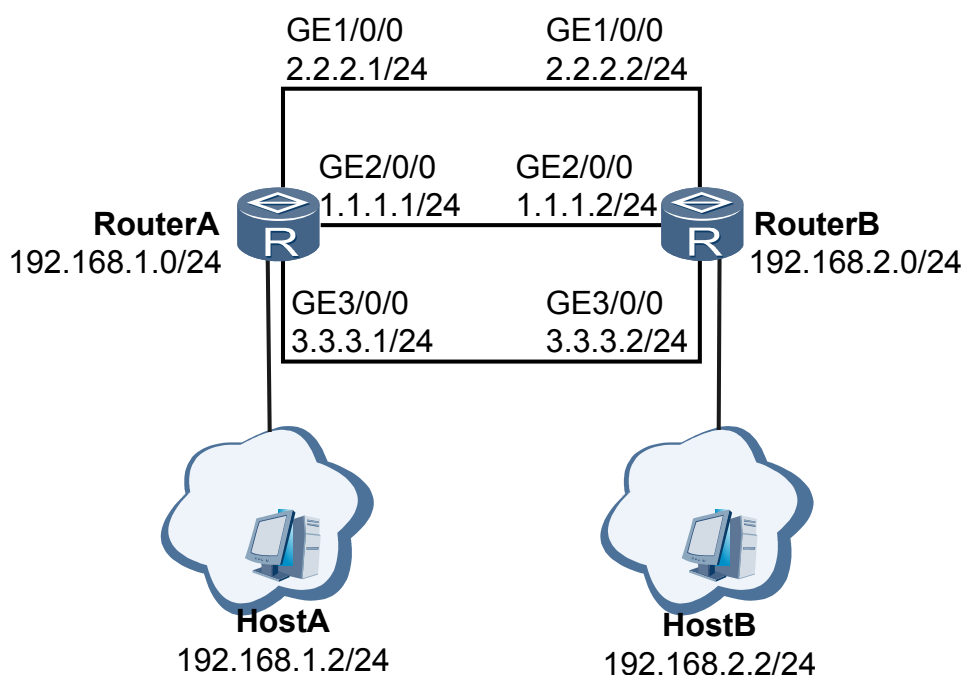
图 1-8 配置负载分担接口备份组网图
