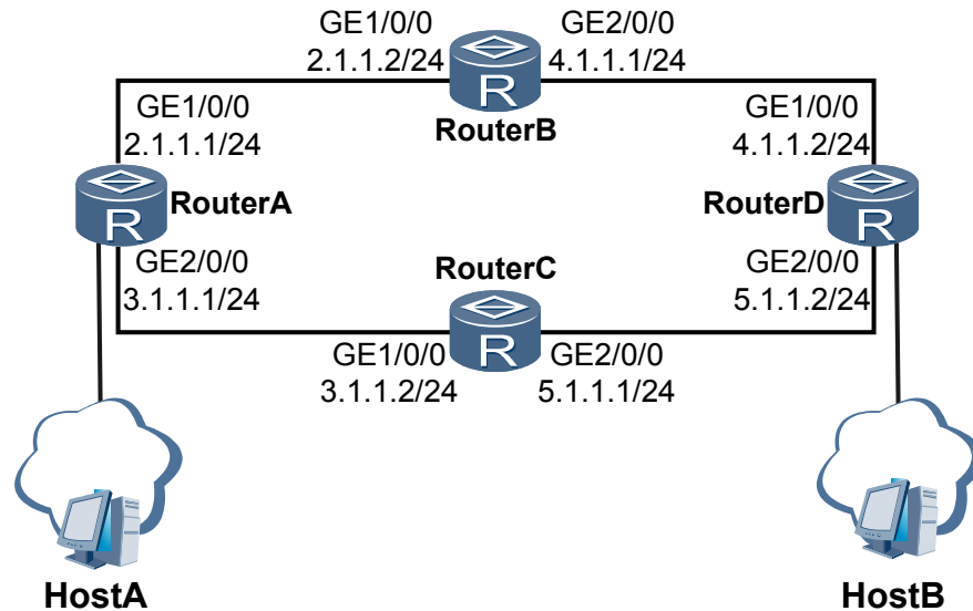
图 1-13 配置接口备份与路由联动组网图
