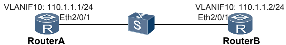
图 3-4 配置 VLANIF 接口单跳检测组网图
