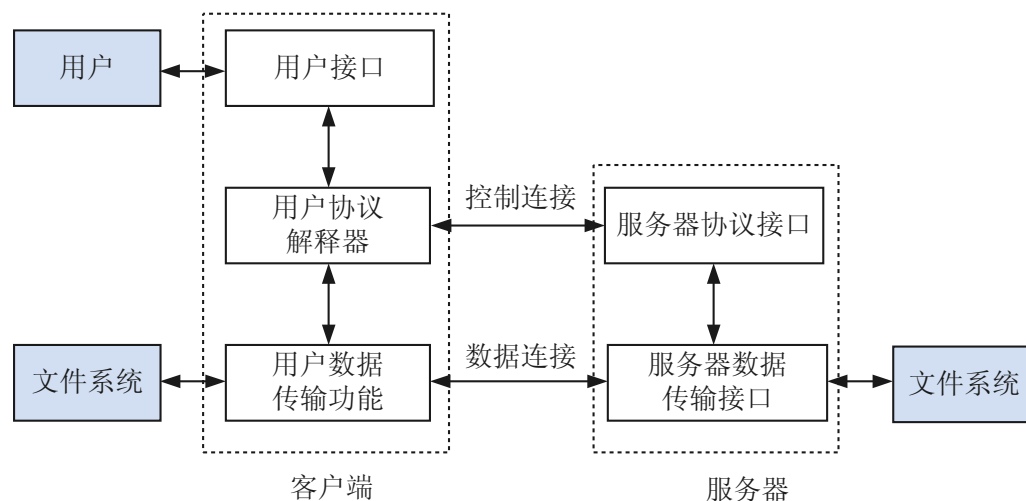
图 1-2 FTP 中的文件传输
