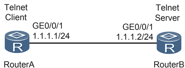
图 1-12 Telnet 登录方式组网图
