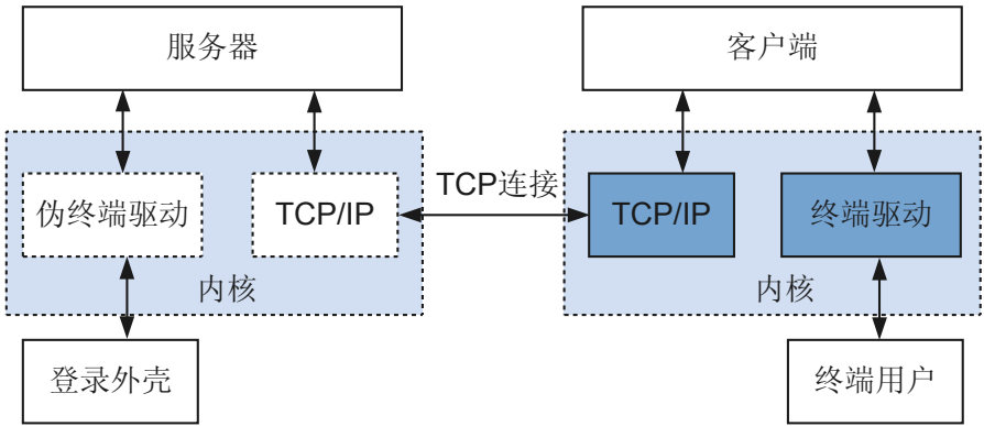
图 1-4 Telnet 连接的示意图
