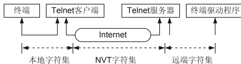
图 1-3 物理终端与 NVT 的转换模型
