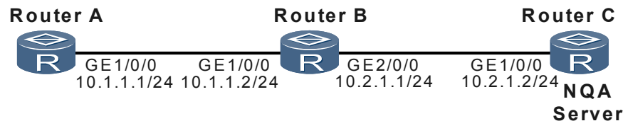
图 5-12 UDP 测试组网图
