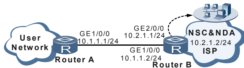
图 6-4 Flexible Netstream 组网图
