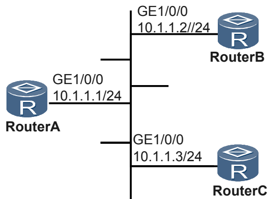
图 4-5 配置 NTP 组播模式的组网图
