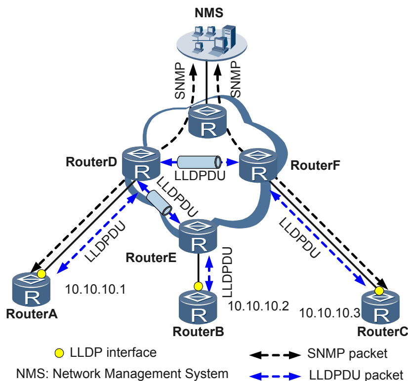
图 2-8 配置 LLDP 功能-多邻居组网图
