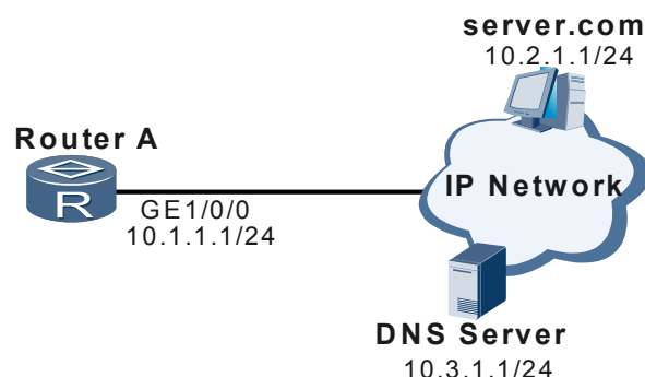
图 5-8 DNS 测试组网图
