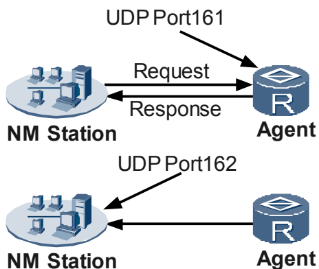
图 1-1 SNMP 结构示意图
