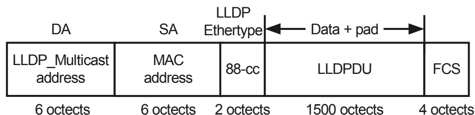
图 2-2 LLDP 报文结构
