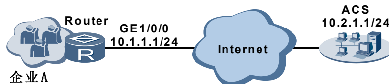
图 3-2 ACS 通过 CWMP 管理 Router
