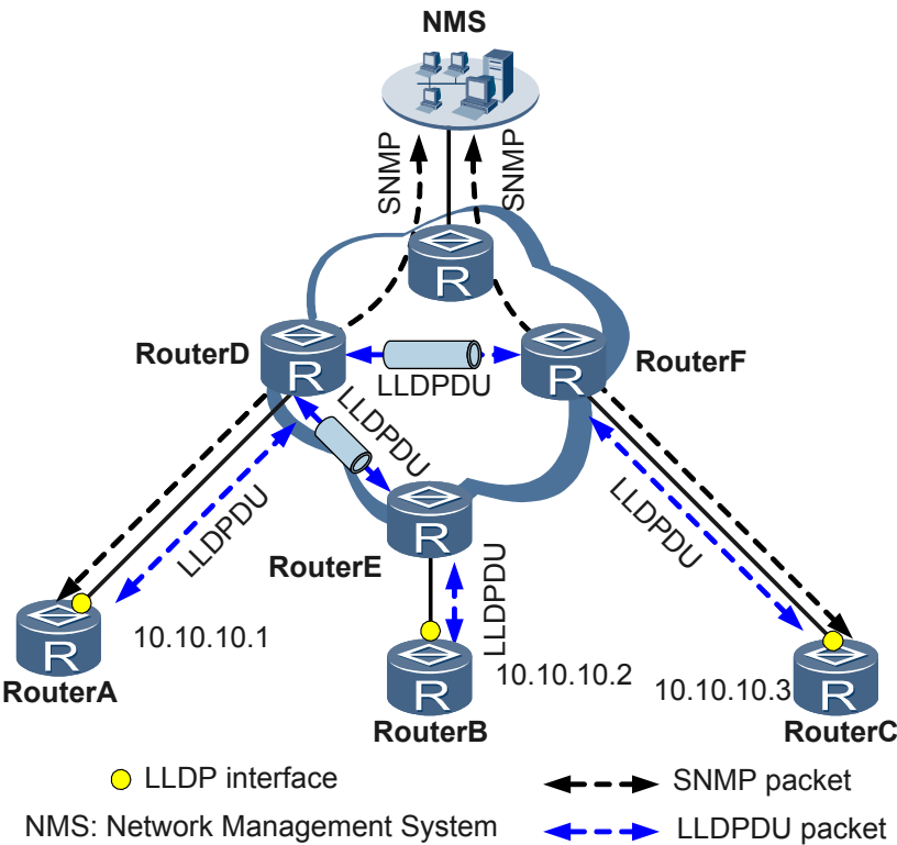
图 2-5 多邻居组网方式
