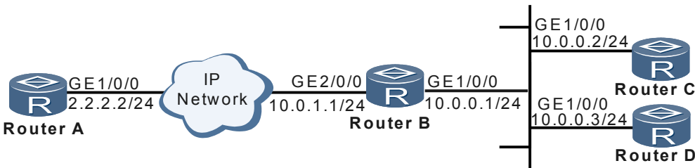
图 4-2 单播 NTP 客户端/服务器模式组网图
