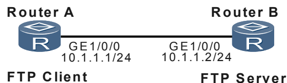
图 5-5 FTP 测试组网图
