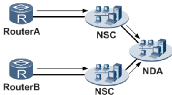
图 6-1 NetStream 数据采集和分析图
