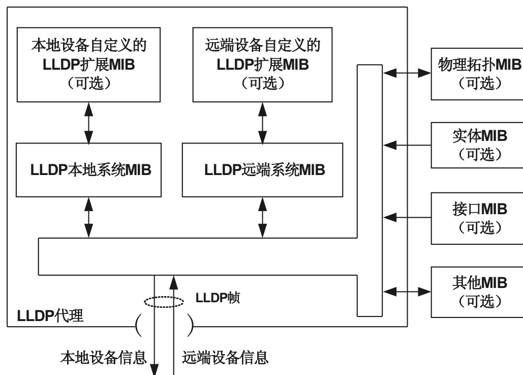
图 2-1 LLDP 结构框图
