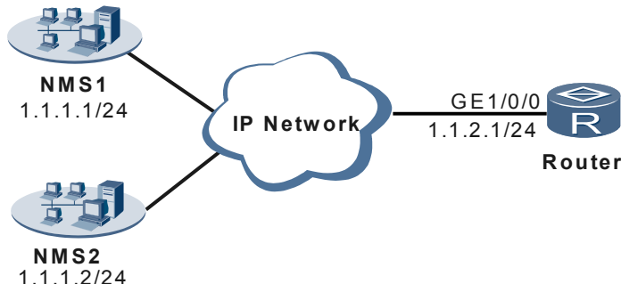
图 1-6 配置使用 SNMPv3 网管通信组网图
