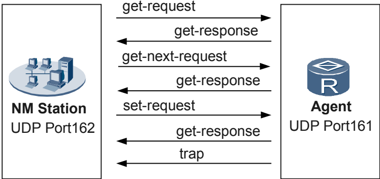
图 1-3 SNMP 操作示意图
