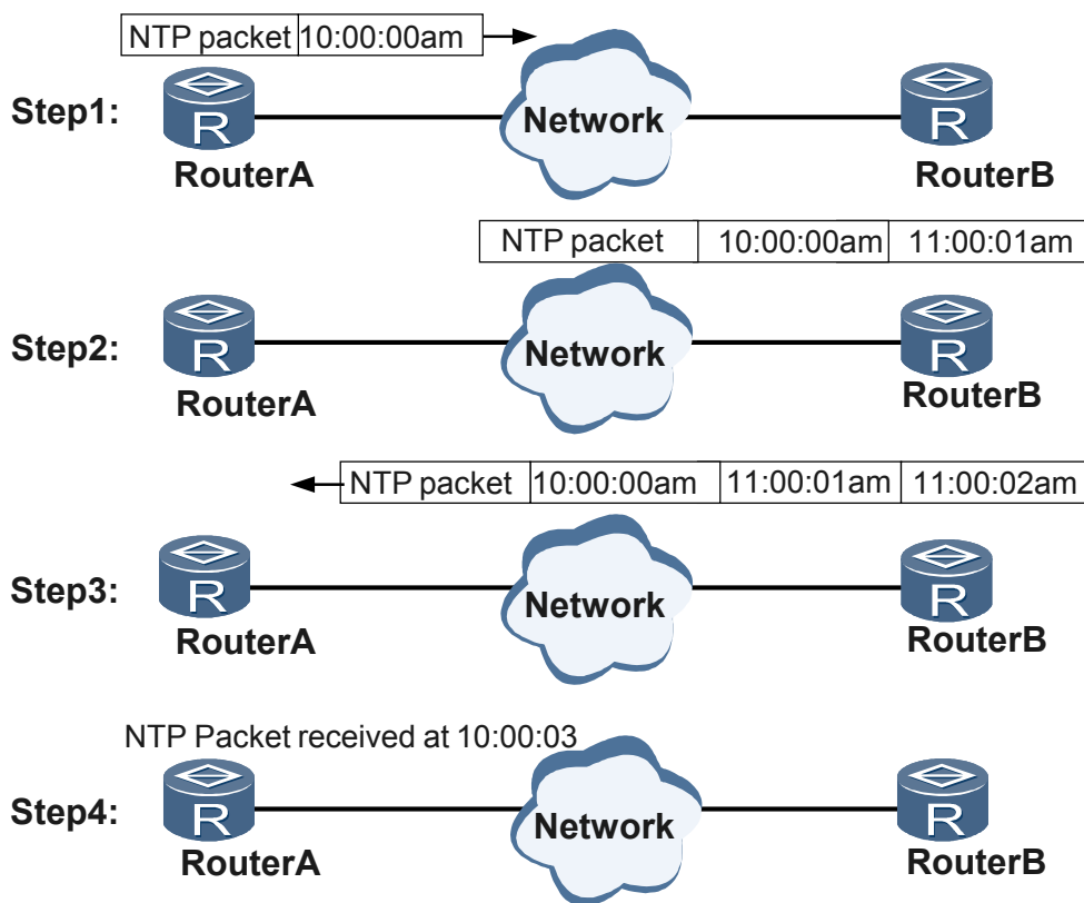
图 4-1 NTP 基本原理图
