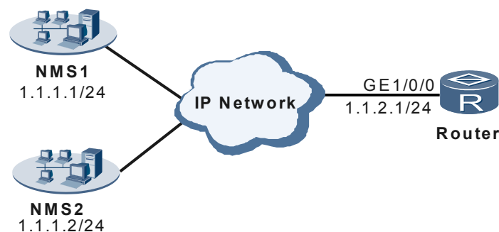
图 1-5 配置使用 SNMPv2c 管通信组网图
