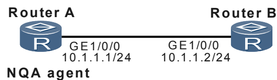
图 5-3 ICMP 测试组网图
