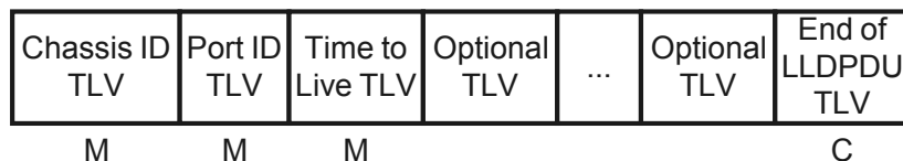
图 2-3 LLDPDU 结构
