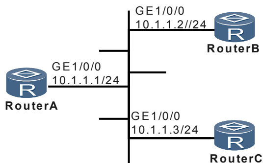
图 4-4 配置 NTP 广播模式的组网图
