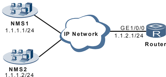
图 1-4 配置使用 SNMPv1 与网管通信组网图
