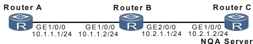
图 5-13 Jitter 测试组网图
