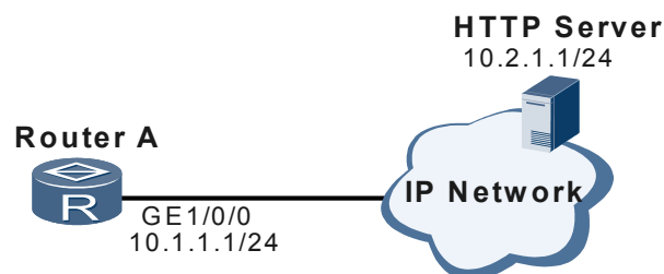
图 5-7 HTTP 测试组网图
