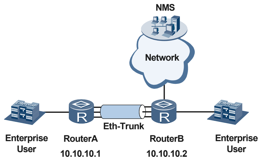
图 2-9 配置 LLDP 功能示例组网图-组网中存在链路聚合
