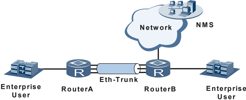
图 2-6 存在链路聚合的组网方式
