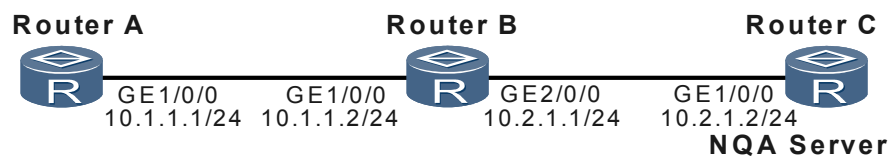
图 5-11 TCP 测试组网图
