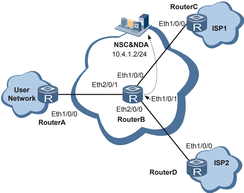
图 6-3 Netstream 聚合组网图
