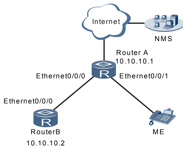
图 2-7 配置 LLDP 功能-单邻居组网图
