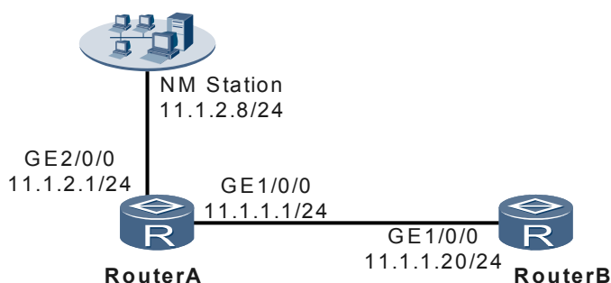
图 5-16 配置 NQA 阈值告警组网图
