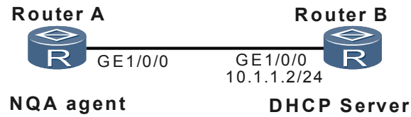
图 5-4 DHCP 测试组网图
