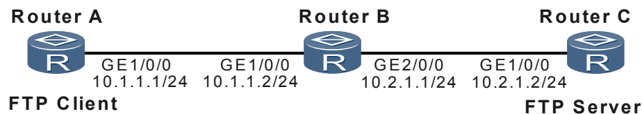
图 5-6 FTP 测试组网图
