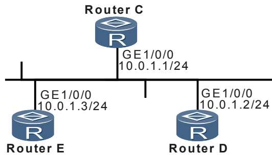
图 4-3 配置 NTP 对等体模式的组网图
