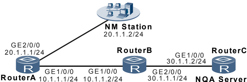
图 5-14 配置 NQA 阈值组网图
