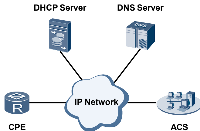
图 3-1 CWMP 网络模型图
