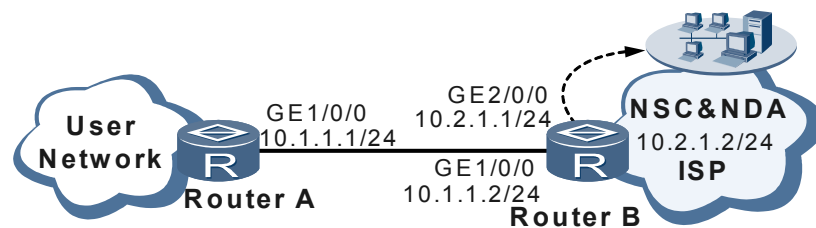
图 6-2 配置 IPv4 单播流量统计组网图
