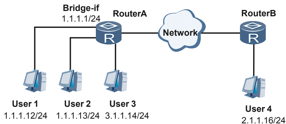
图 2-3 透明网桥集成路由桥接应用组网图
