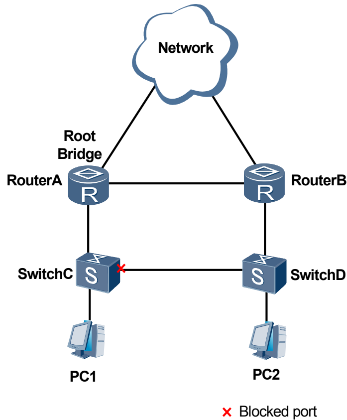
图 7-2 环形网络示意图
