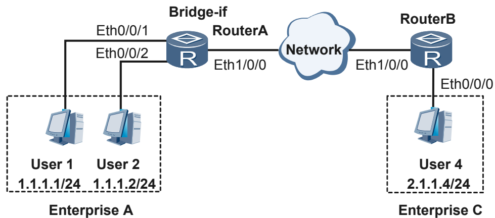
图 2-11 远程不同网段桥接功能组网图
