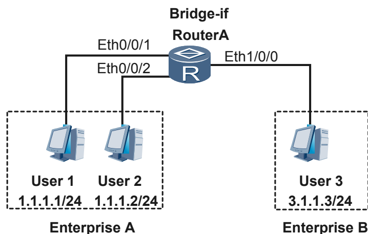
图 2-9 本地不同网段桥接功能组网图
