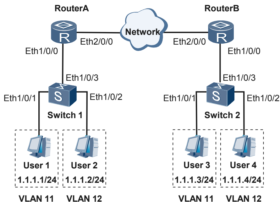
图 2-12 远程桥接组网图
