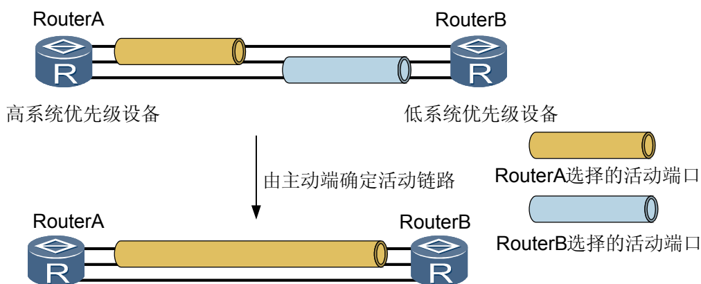
图 1-1 静态 LACP 模式下主动端确定活动链路
