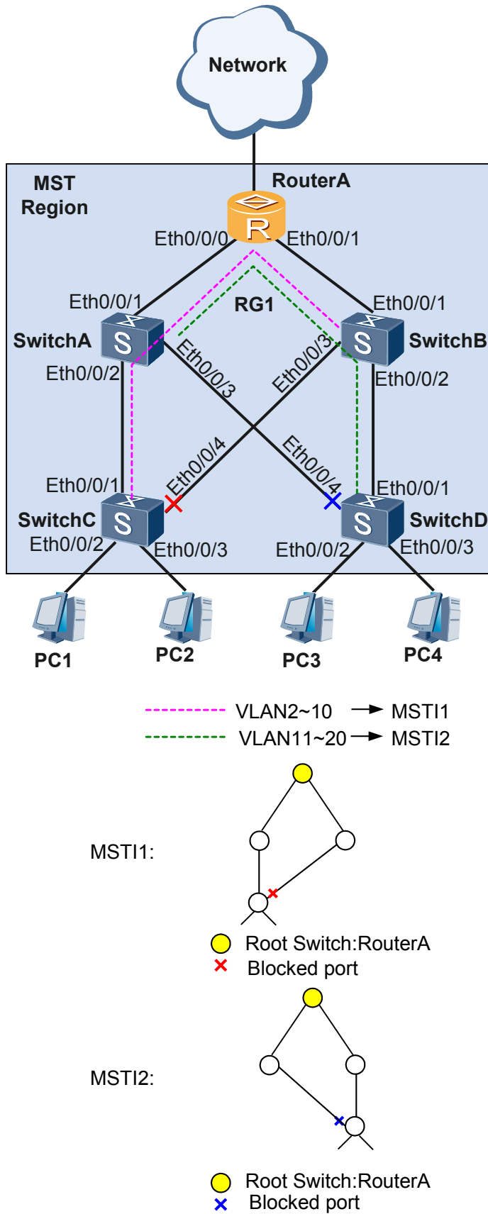
图 8-7 配置 MSTP 功能组网图
