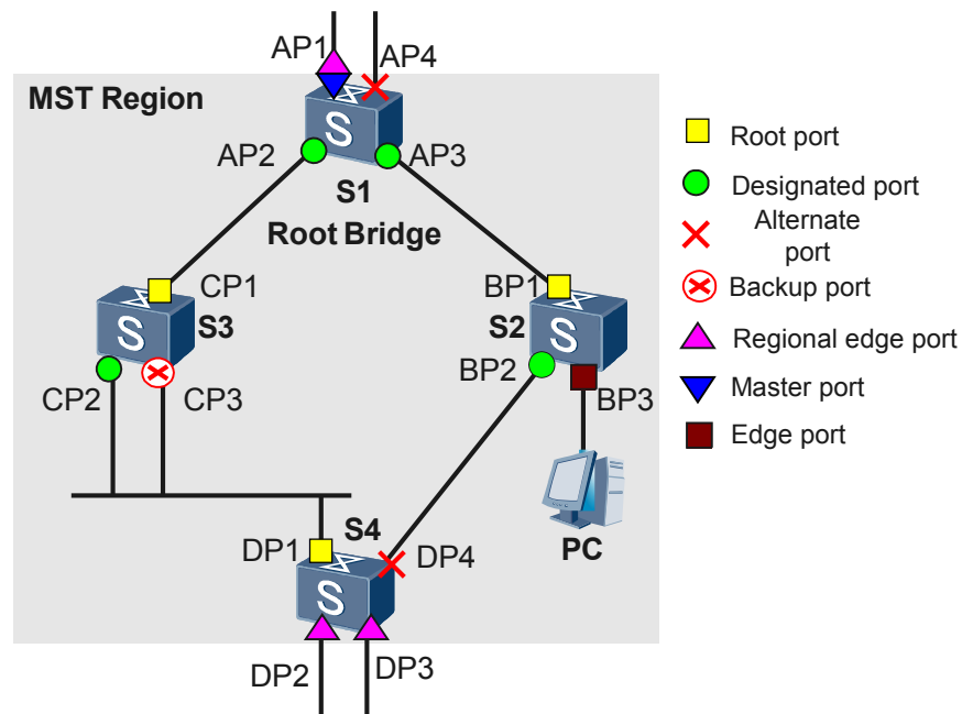
图 8-5 端口角色示意图
