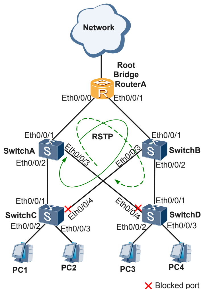
图 7-4 配置 RSTP 功能组网图
