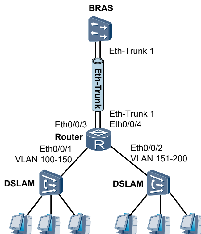
图 1-4 配置手工负载分担模式链路聚合组网图
