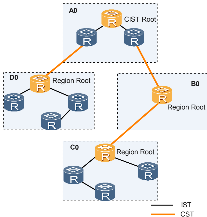
图 8-4 MSTP 网络基本概念示意图
