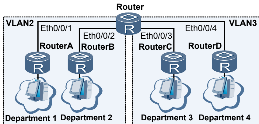
图 3-2 配置基于接口划分 VLAN 组网图
