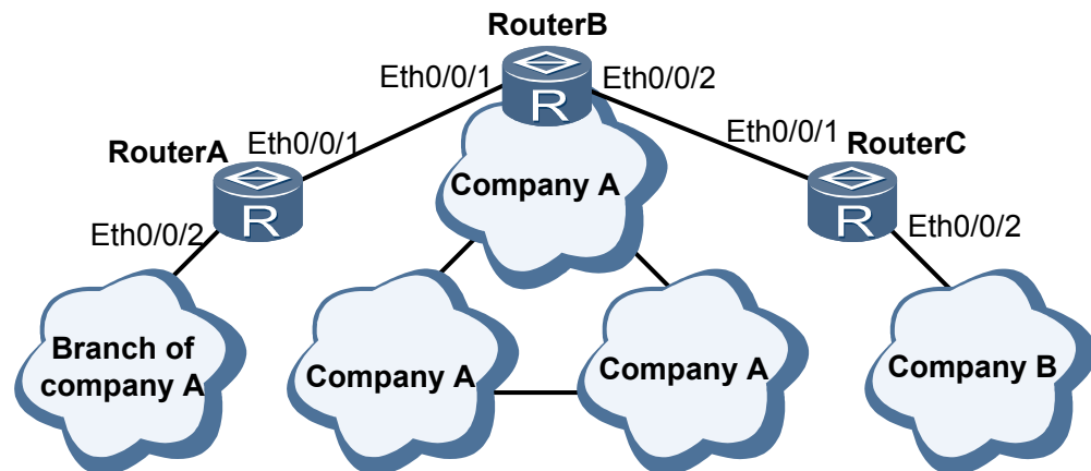
图 5-2 配置 GVRP 的组网图
