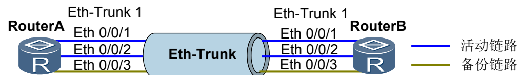
图 1-5 配置静态 LACP 模式链路聚合组网图
