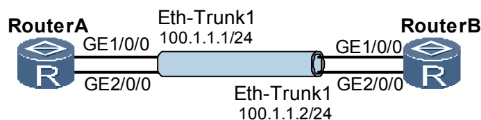
图 1-6 配置三层链路聚合组网图
