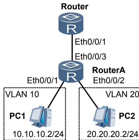
图 3-3 配置 VLAN 间通过 VLANIF 接口通信组网图
