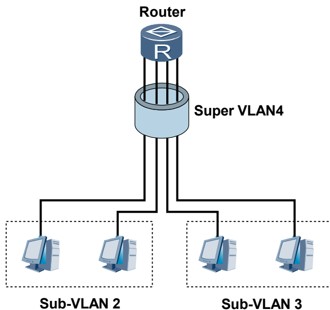
图 3-1 VLAN 聚合应用场景图
