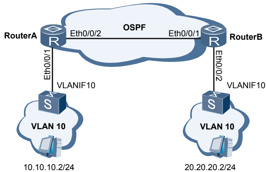
图 3-6 配置通过 VLANIF 接口跨越三层网络通信组网图
