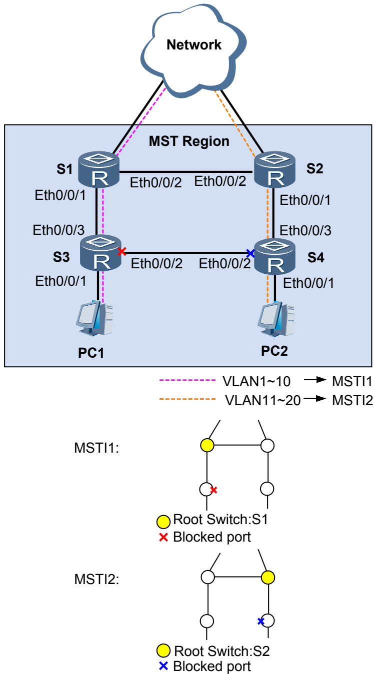
图 8-6 配置 MSTP 的基本功能组网图
