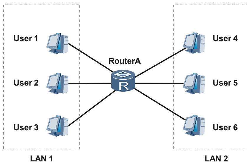
图 2-1 透明网桥本地桥接应用组网图
