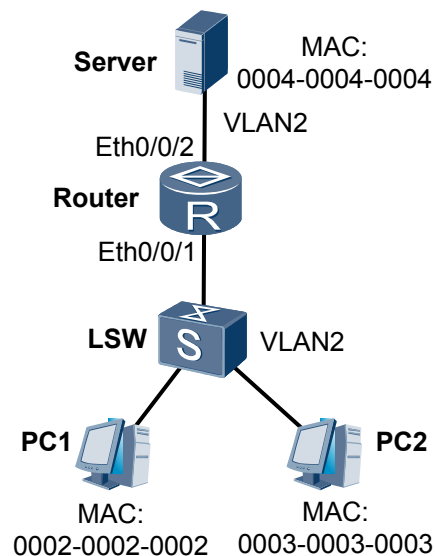
图 6-1 配置 MAC 表组网图
