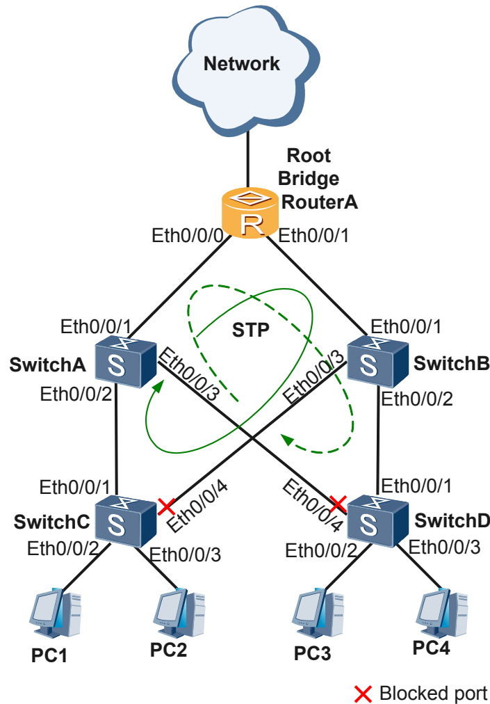
图 7-3 配置 STP 功能组网图
