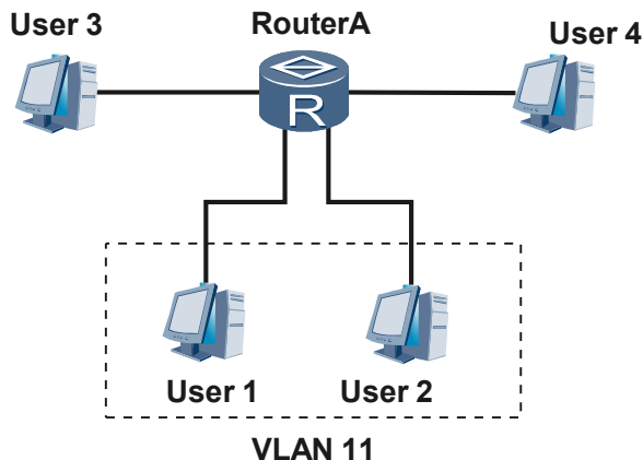
图 2-5 用户加入网桥组方式
