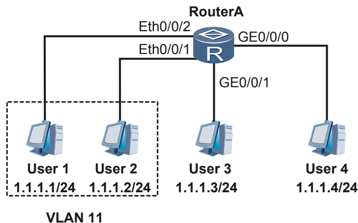
图 2-8 本地同一网段桥接功能示例组网图
