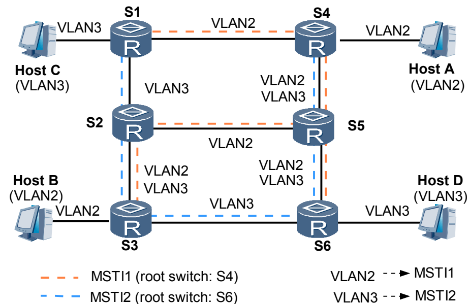
图 8-1 MST 域内的多棵生成树示意图
