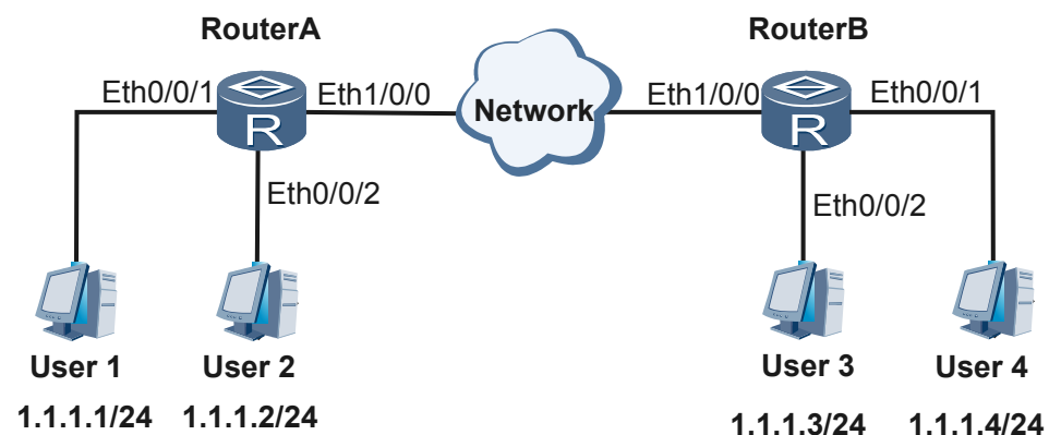
图 2-10 远程同一网段桥接功能组网图
