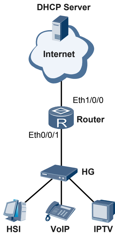
图 4-2 配置手动模式下的 Voice VLAN 的组网图
