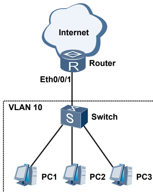
图 6-2 配置接口安全示例组网图
