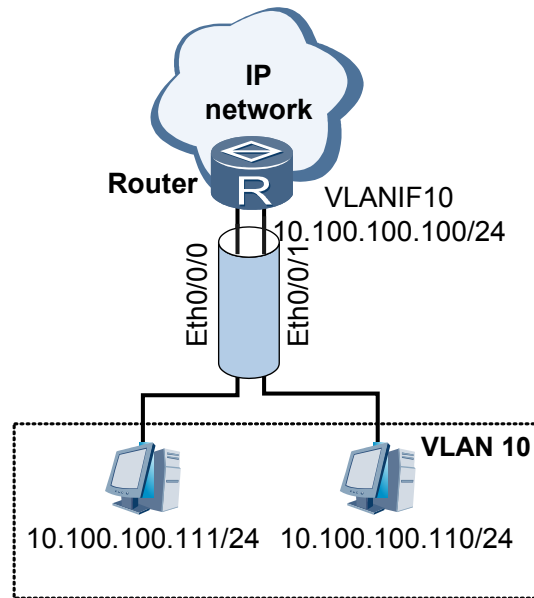
图 3-4 配置 VLAN Damping 组网图
