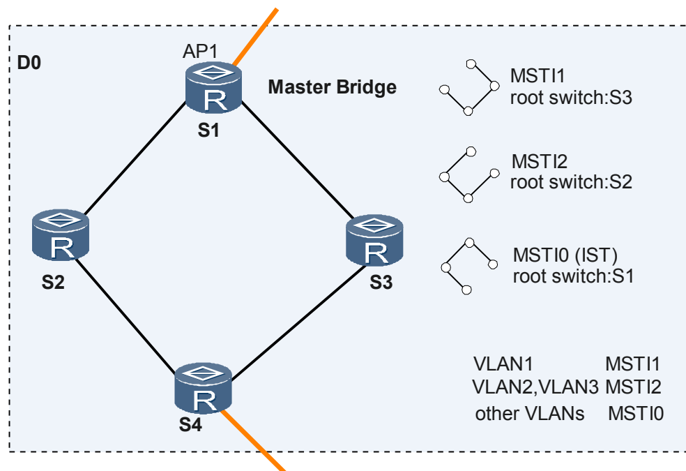
图 8-2 MST Region 的基本概念示意图
