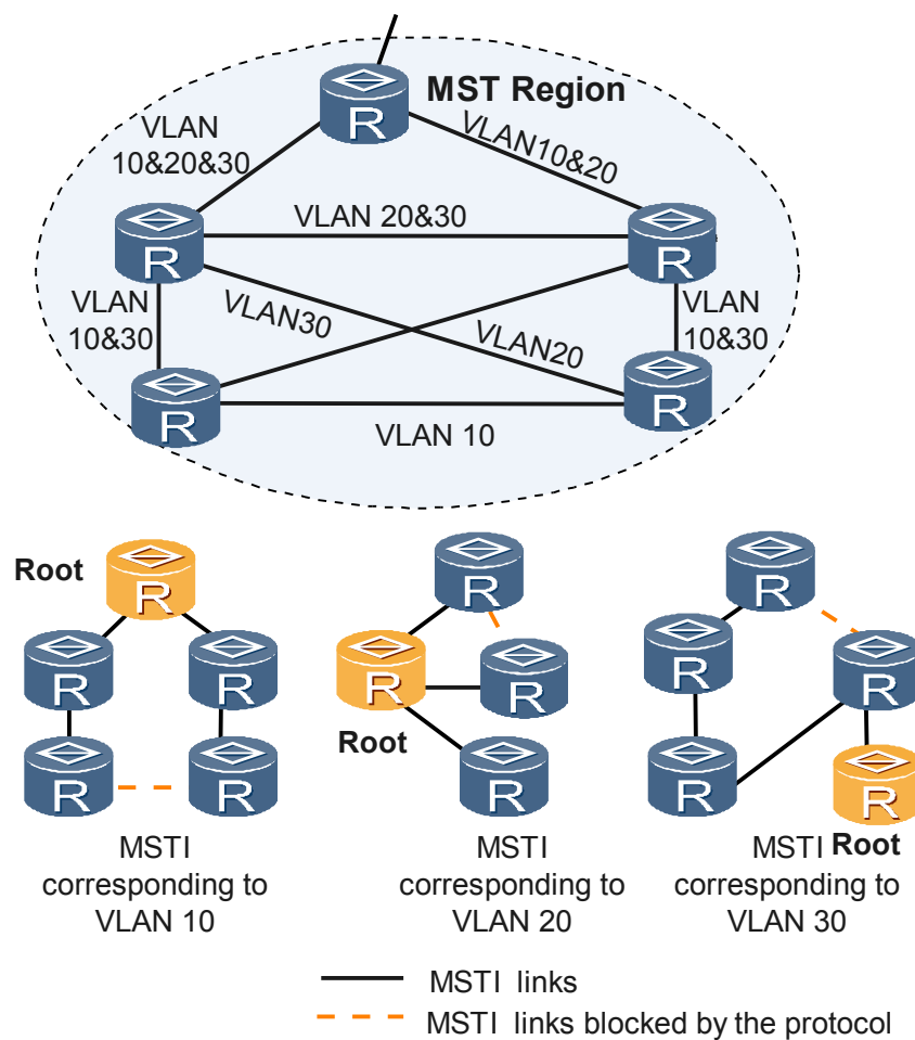
图 8-3 MSTI 的基本概念示意图
