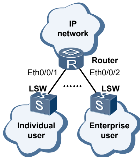
图 6-3 配置基于接口的 MAC 地址学习限制组网图
