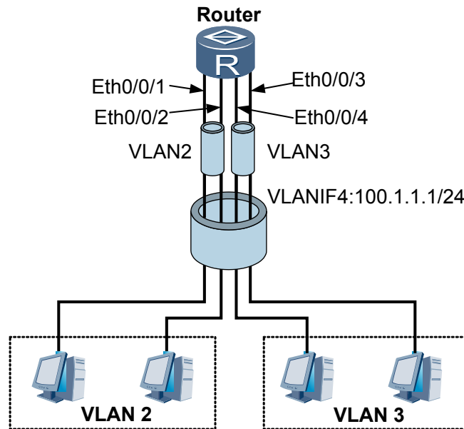
图 3-5 配置 VLAN 聚合组网图
