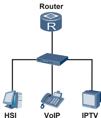
图 3-12 Voice VLAN 组网图
