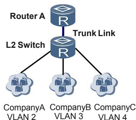
图 3-15 多个 VLAN 属于同一个三层设备互通组网图
