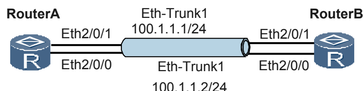
图 1-12 Eth-Trunk 组网图
