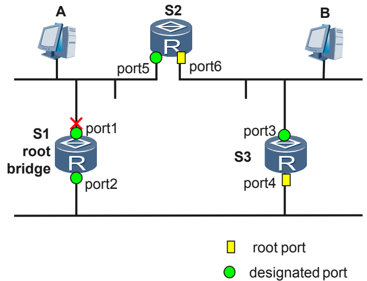
图 5-14 拓扑变化示意图-根桥指定端口发生故障
