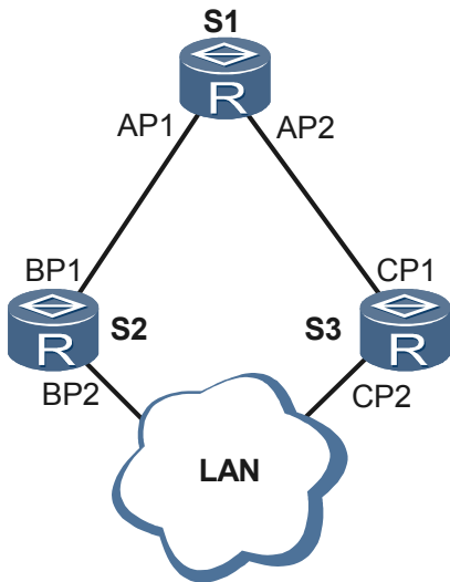
图 5-3 指定桥与指定端口示意图
