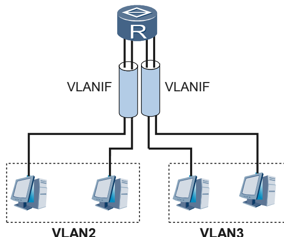
图 3-6 通过三层交换机实现 VLAN 间的通信
