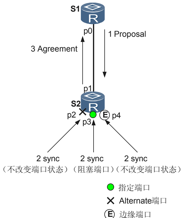
图 5-18 Proposal/Agreement 过程示意图
