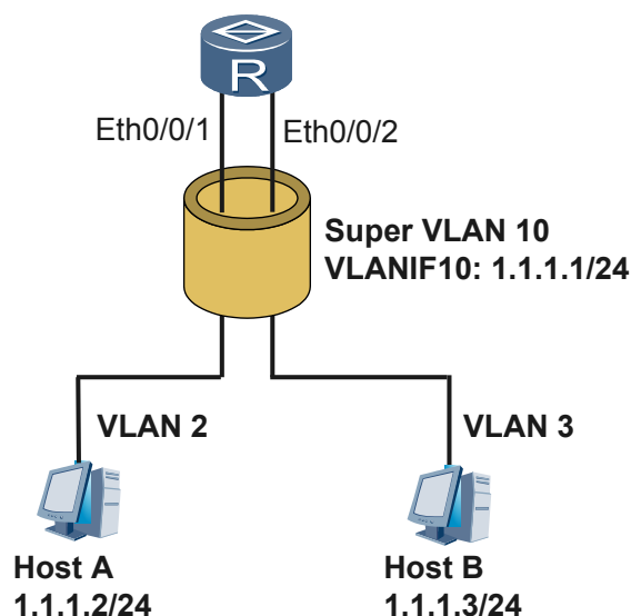
图 3-9 ARP Proxy 实现不同 sub-VLAN 间的三层互通组网图
