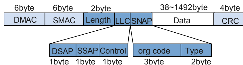
图 5-6 以太网数据帧格式
