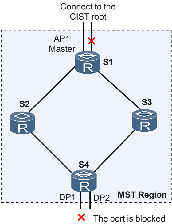
图 5-26 Master 端口和域边缘端口示意图
