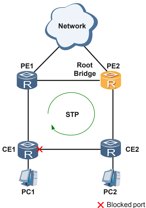
图 5-31 STP 典型应用组网图
