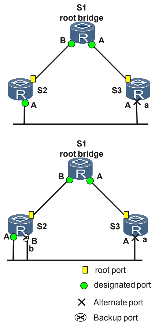
图 5-15 端口角色示意图
