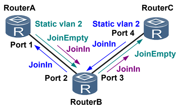
图 4-6 VLAN 属性的双向注册
