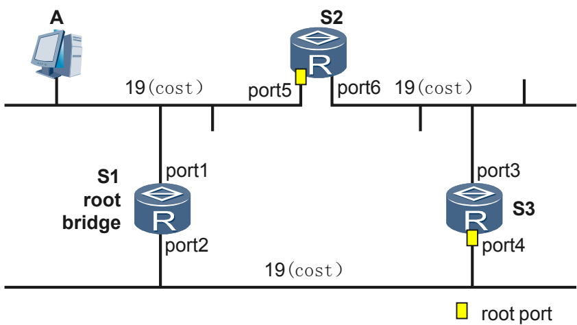
图 5-10 根端口选举示意图
