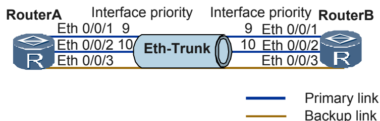
图 1-11 LACP 抢占场景
