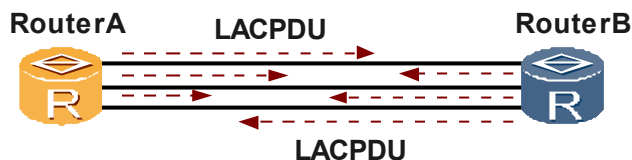
图 1-8 静态 LACP 模式链路聚合互发 LACPDU
