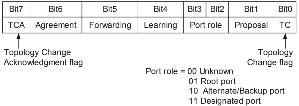
图 5-16 RSTP Flag 字段格式
