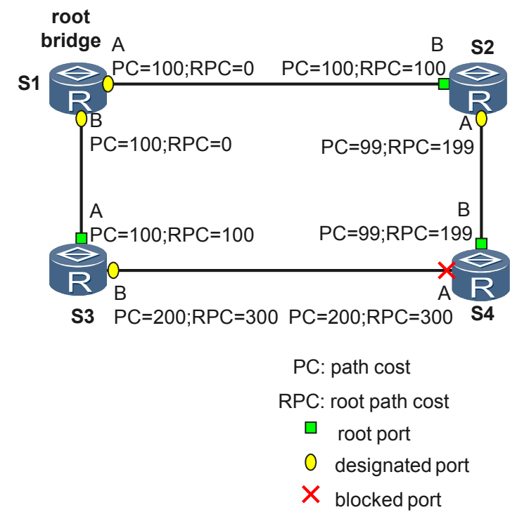
图 5-2 STP 网络结构
