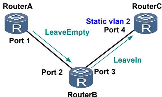
图 4-7 VLAN 属性的单向注销
