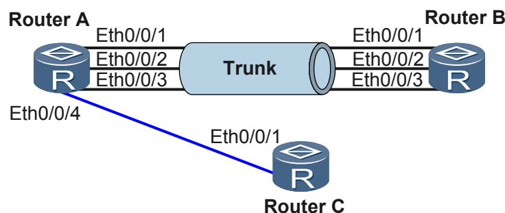
图 1-4 Trunk 错连示意图
