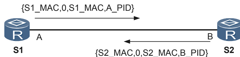
图 5-8 初始信息交互
