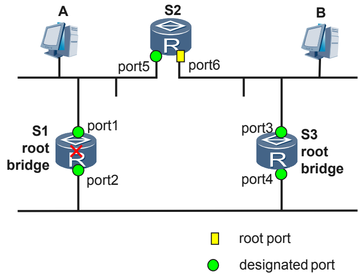
图 5-13 拓扑变化示意图-根桥发生故障
