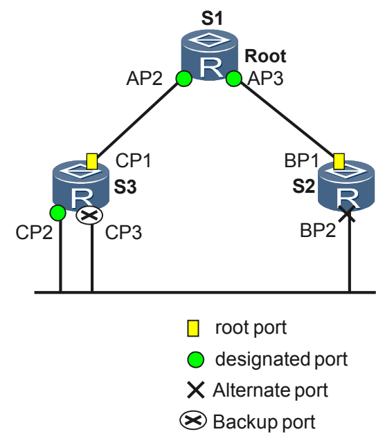
图 5-25 根端口、指定端口、Alternate 端口和 Backup 端口示意图
