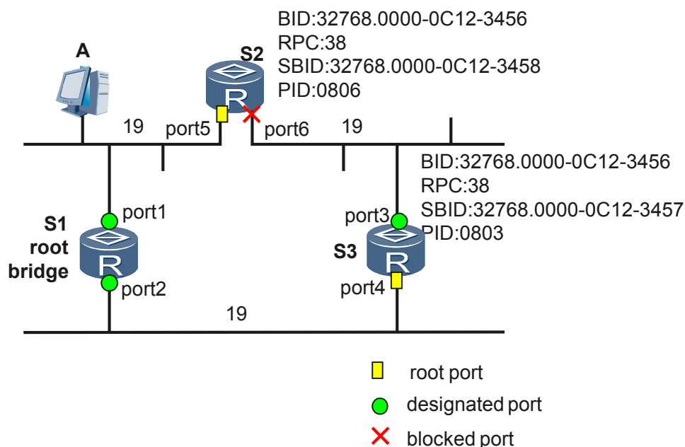
图 5-11 指定端口选举示意图
