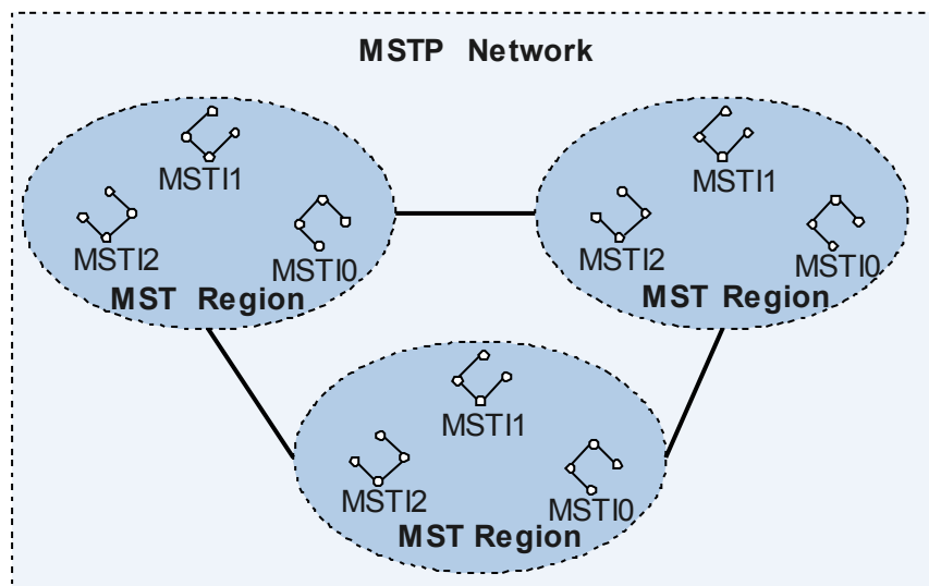
图 5-21 MSTP 网络层次示意图
