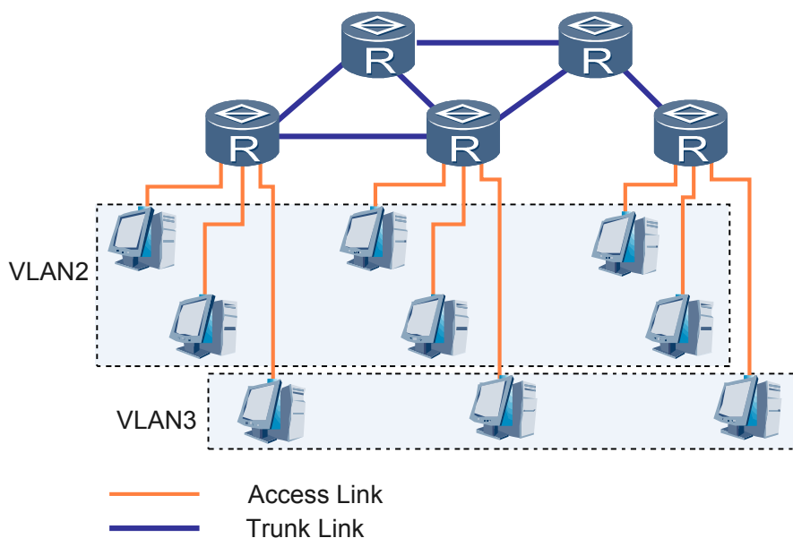
图 3-3 链路类型示意图
