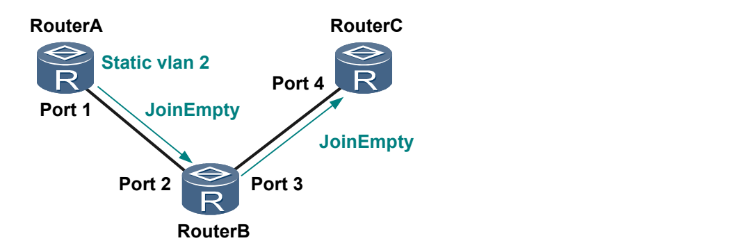
图 4-5 VLAN 属性的单向注册
