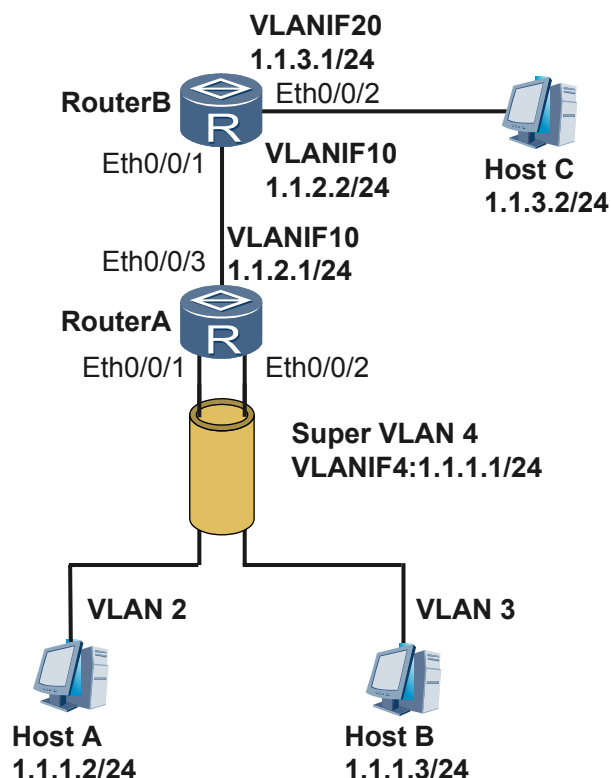
图 3-11 sub-VLAN 与外部网络的三层通信组网图
