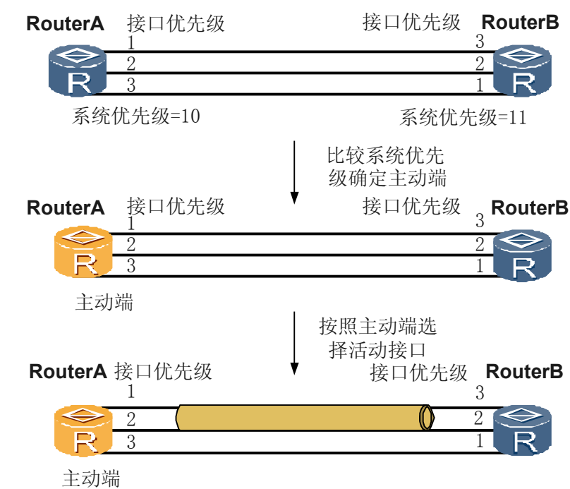
图 1-10 静态 LACP 模式选择活动接口的过程
