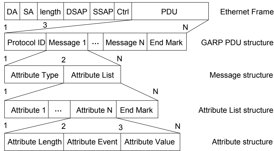
图 4-4 GARP 协议报文
