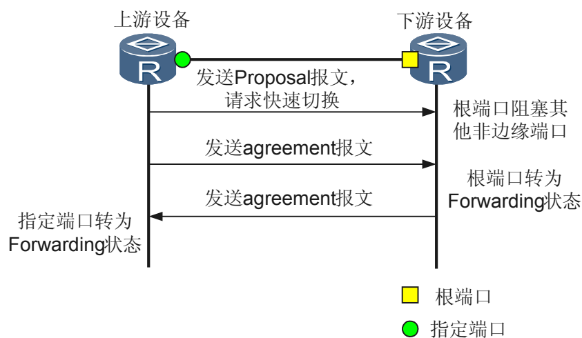
图 5-30 增强方式的 P/A 机制
