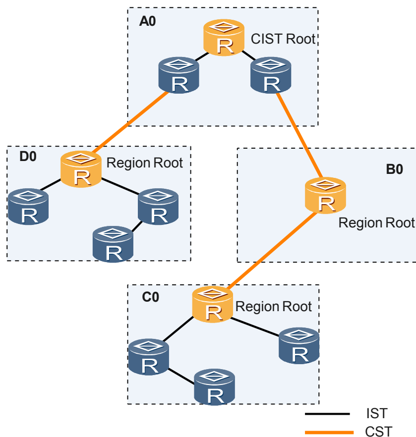
图 5-24 MSTP 网络基本概念示意图
