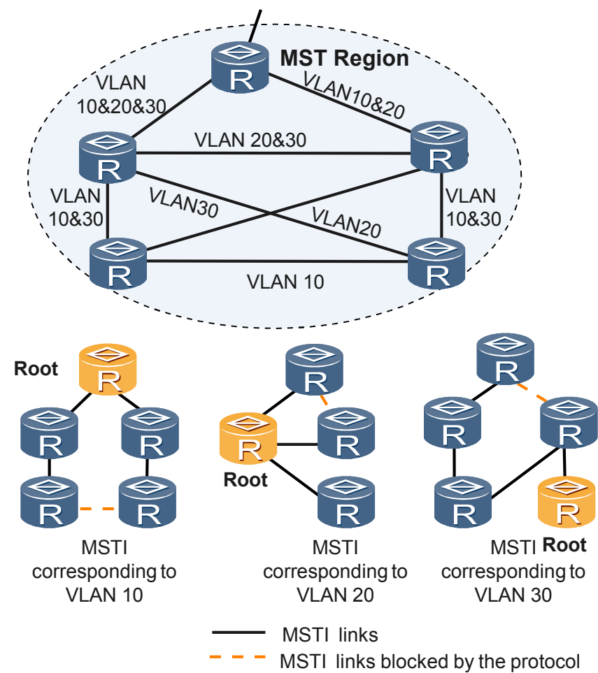
图 5-23 MSTI 的基本概念示意图
