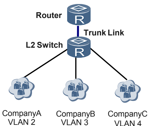
图 3-13 基于端口的 VLAN 划分组网图
