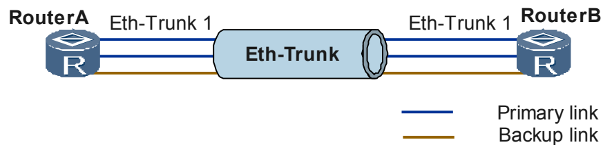
图 1-5 M:N 备份示意图
