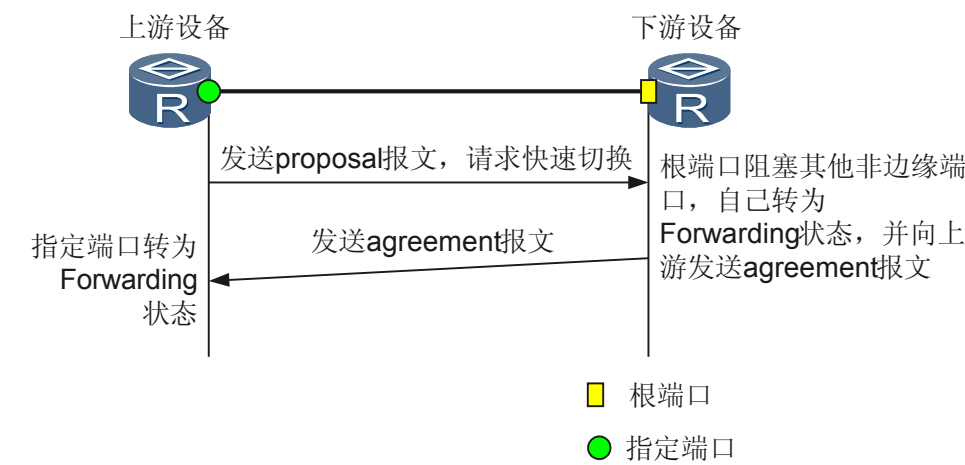
图 5-17 Proposal/ Agreement 过程示意图
