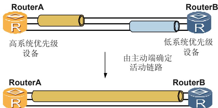
图 1-9 确定静态 LACP 模式主动端
