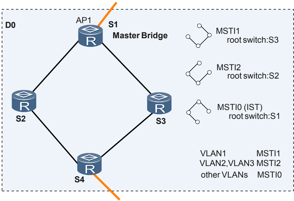
图 5-22 MST Region 的基本概念示意图
