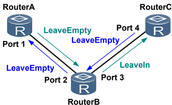
图 4-8 VLAN 属性的双向注销
