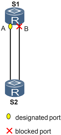
图 5-4 应用到 PID 进行比较的拓扑
