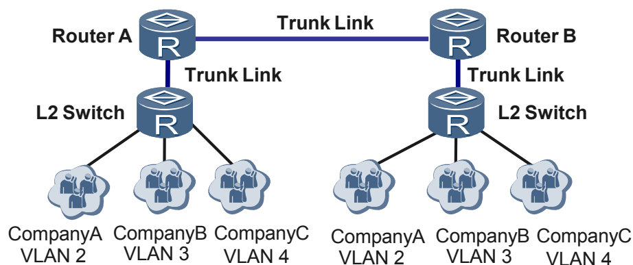
图 3-16 多个 VLAN 跨越三层设备互通组网图
