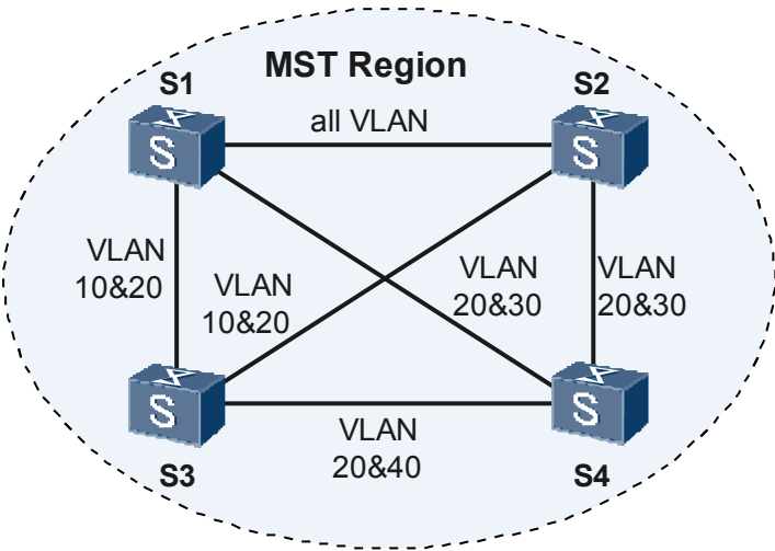
图 5-32 MSTP 典型应用组网图
