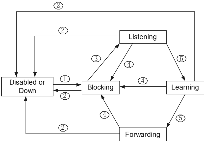
图 5-5 端口状态迁移图
