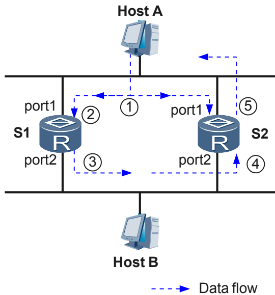
图 5-1 典型局域网络示意图
