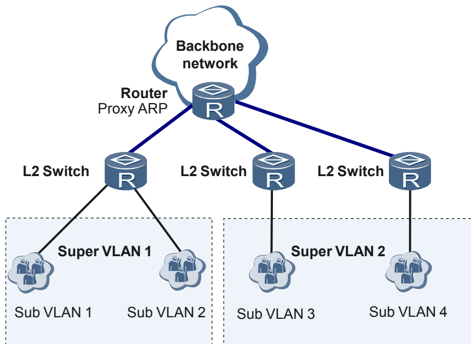
图 3-17 VLAN Aggregation 应用组网图
