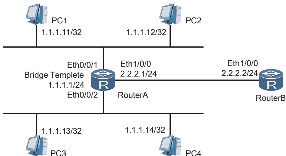
图 2-3 透明网桥集成路由桥接应用
