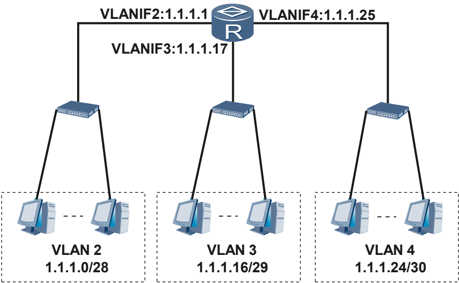
图 3-7 普通 VLAN 网络示意图
