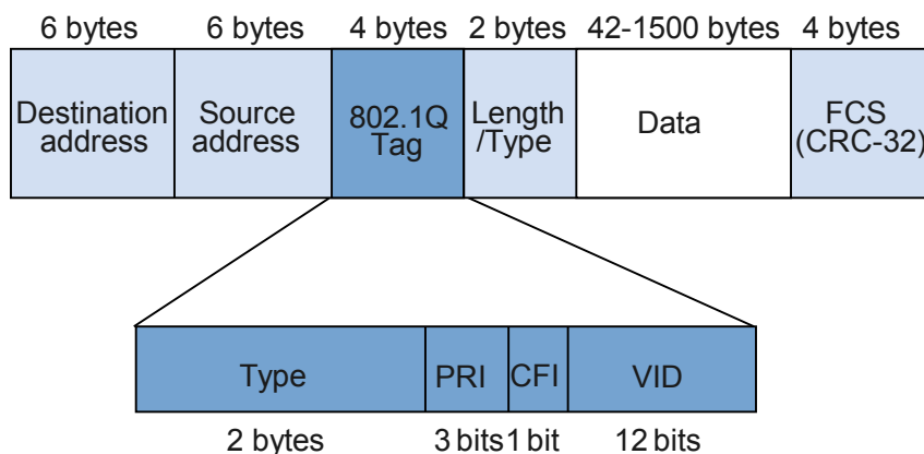
图 3-2 基于 802.1Q 的 VLAN 帧格式
