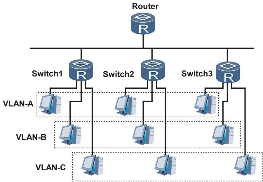
图 3-1 VLAN 的典型应用示意图
