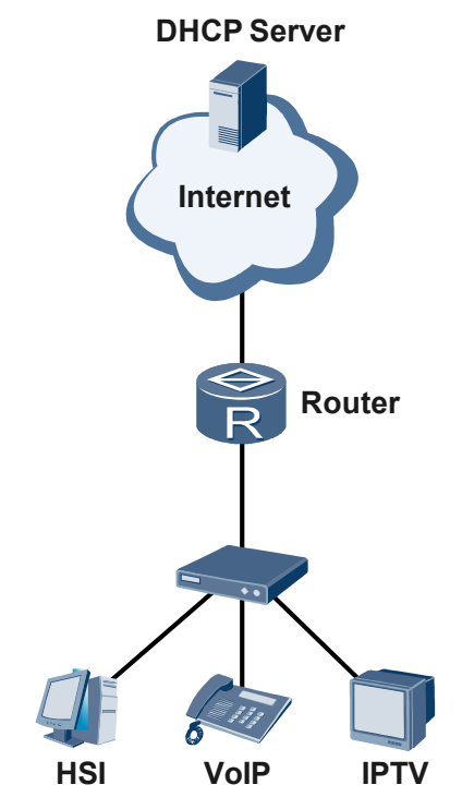
图 3-18 Voice VLAN 的应用组网图
