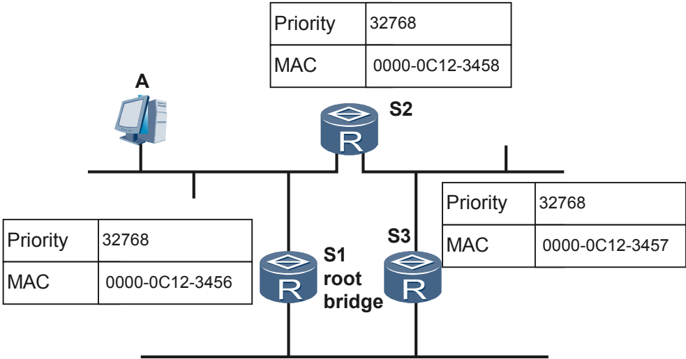
图 5-9 根桥选举示意图
