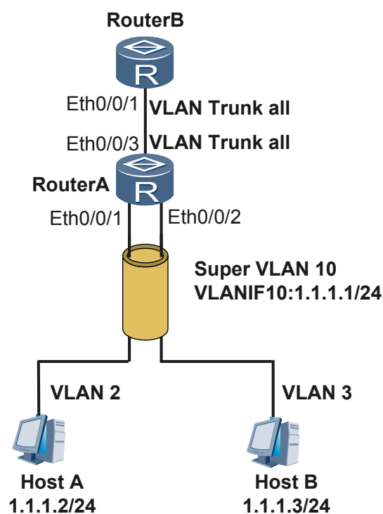
图 3-10 sub-VLAN 与外部网络的二层通信组网图
