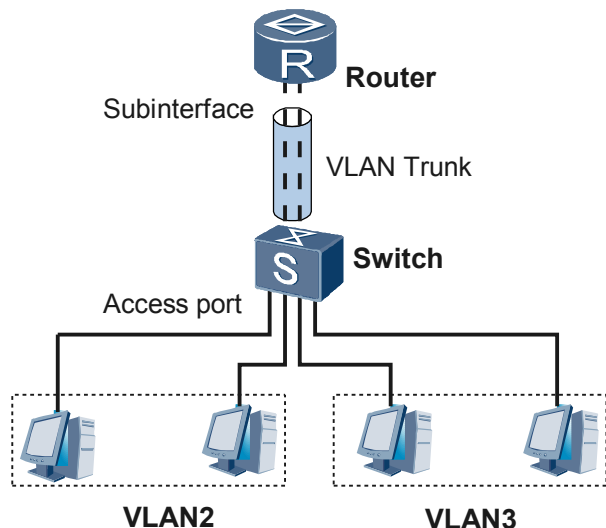
图 3-5 通过二层交换机+路由器实现 VLAN 间的通信
