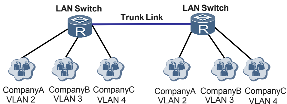
图 3-14 VLAN Trunk 的应用组网图
