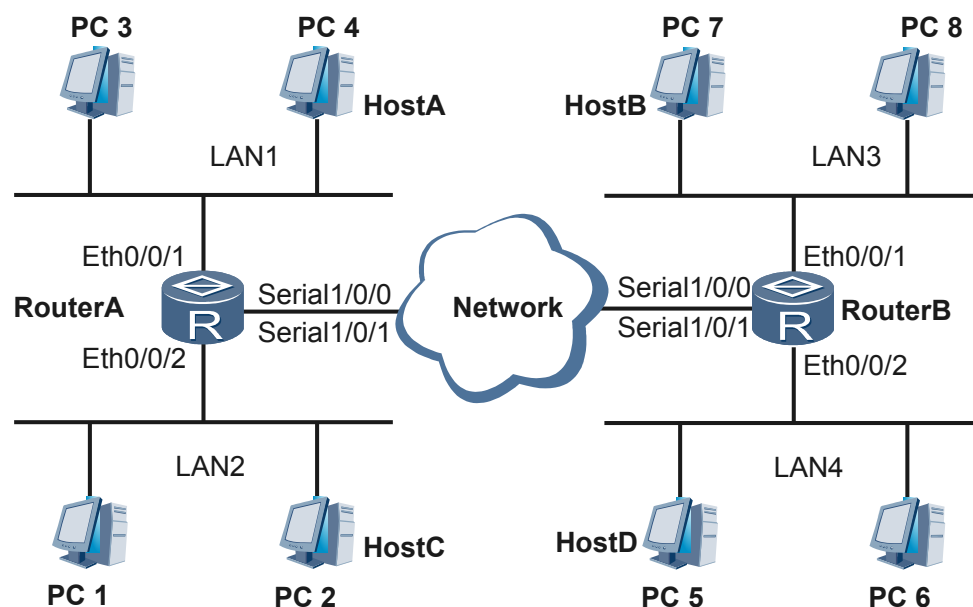
图 2-2 透明网桥远程桥接应用
