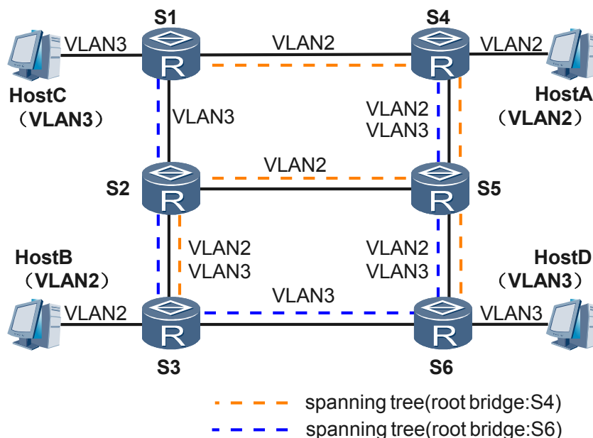
图 5-20 MST 域内的多棵生成树示意图
