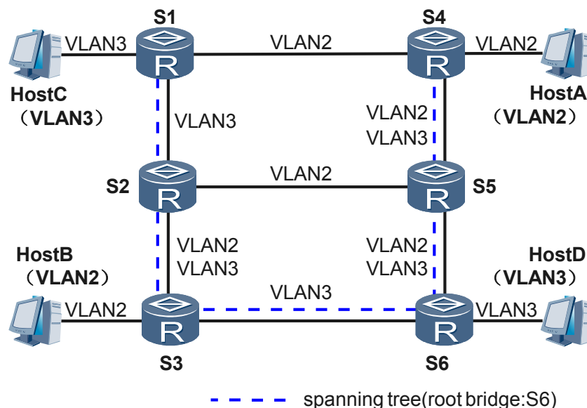
图 5-19 STP/RSTP 的缺陷示意图
