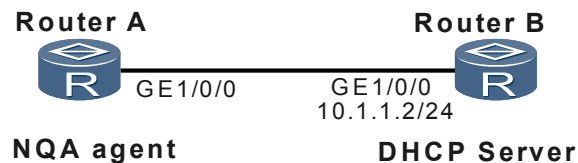
图 5-4 DHCP 测试组网图
