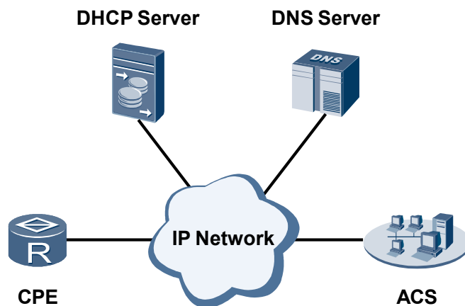
图 3-1 CWMP 网络模型图
