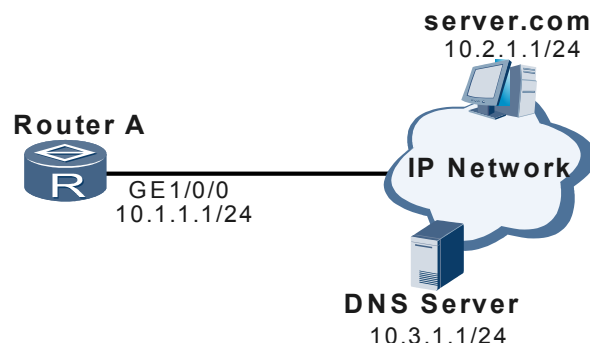
图 5-8 DNS 测试组网图
