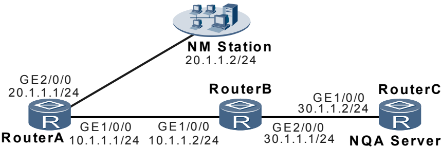
图 5-14 配置 NQA 阈值组网图
