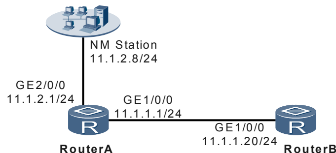
图 5-16 配置 NQA 阈值告警组网图
