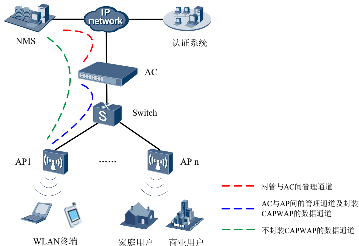
图 1-1 Fit AP 典型组网图(接入点模式)
