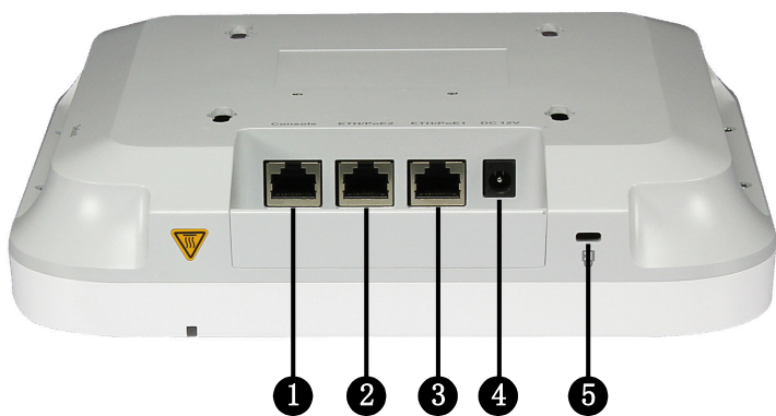
图 2-2 AP7130DN-AC 端口图
