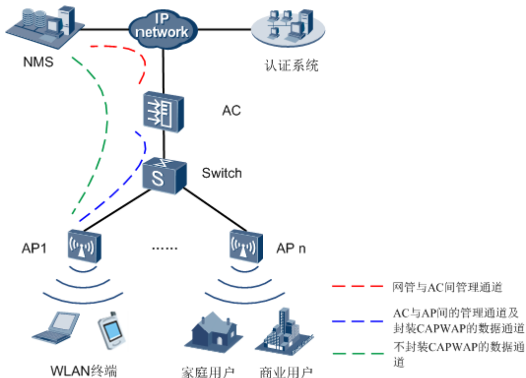
图 1-1 Fit AP 典型组网图(接入点模式)
