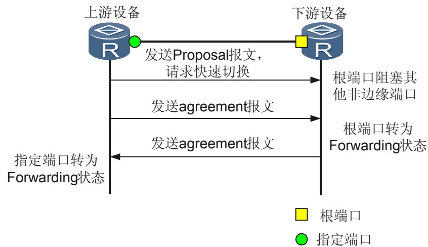
图 5-29 增强方式的 P/A 机制
