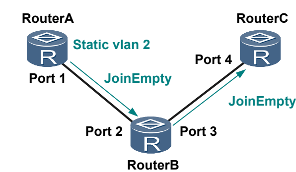
图 4-5 VLAN 属性的单向注册
