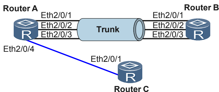
图 1-4 Trunk 错连示意图
