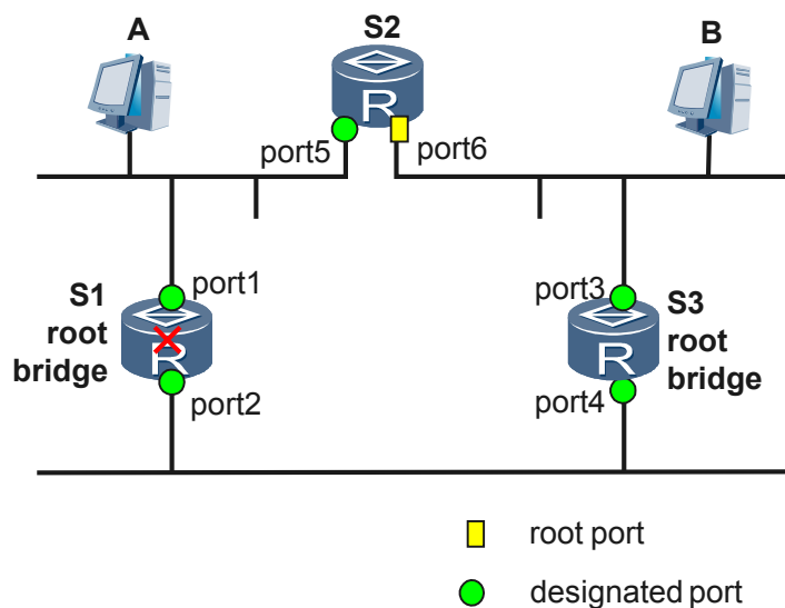
图 5-13 拓扑变化示意图-根桥发生故障
