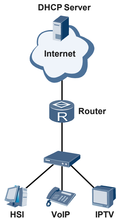
图 3-18 Voice VLAN 的应用组网图
