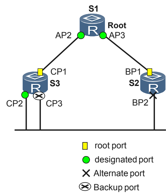
图 5-25 端口角色示意图
