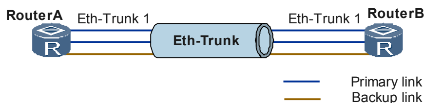
图 1-5 M:N 备份示意图
