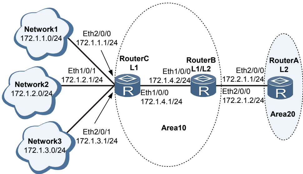
图 7-4 配置 IS-IS 的路由聚合组网图
