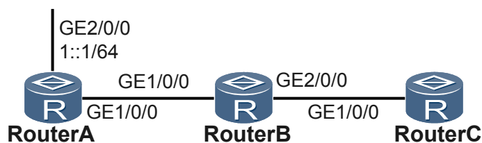
图 4-1 配置 RIPng 基本功能组网图
