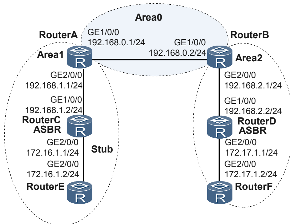
图 5-8 配置 OSPF Stub 区域组网图
