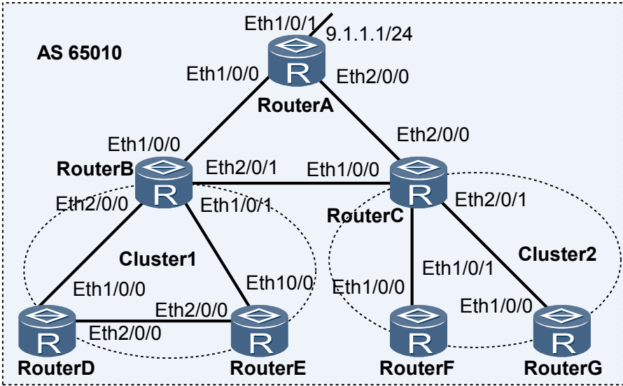
图 8-9 配置 BGP 路由反射器组网图
