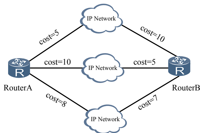
图 5-4 等价路由组网图
