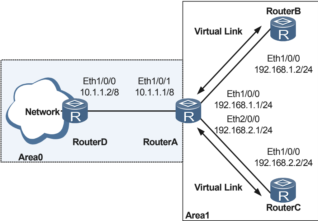
图 5-12 OSPF GTSM 组网图
