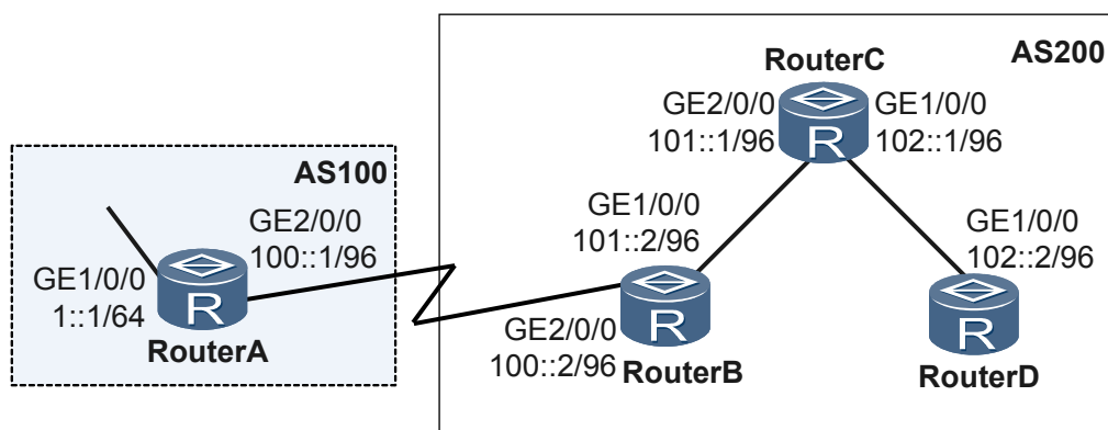
图 9-2 配置 BGP 路由反射器组网图
