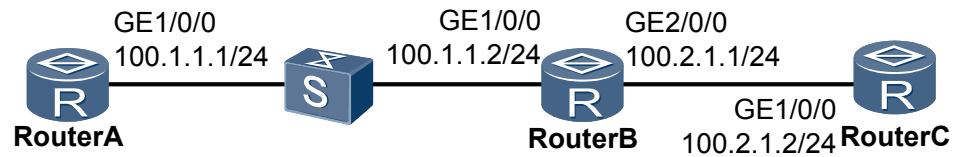
图 7-11 配置静态 BFD for IS-IS 组网图
