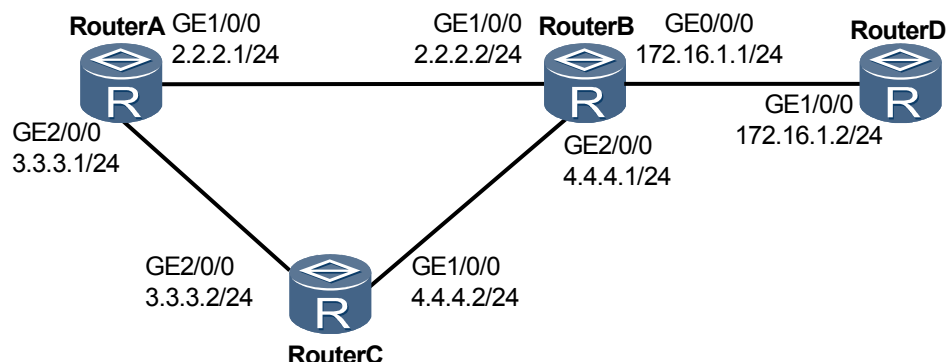
图 3-3 配置静态 BFD for RIP 组网图
