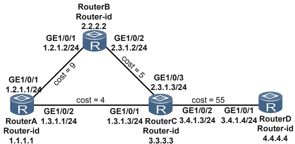
图 5-10 配置 OSPF IP FRR 组网图
