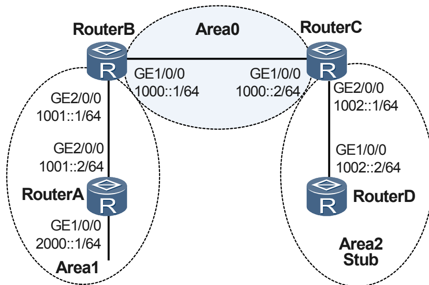
图 6-1 配置 OSPFv3 区域组网图
