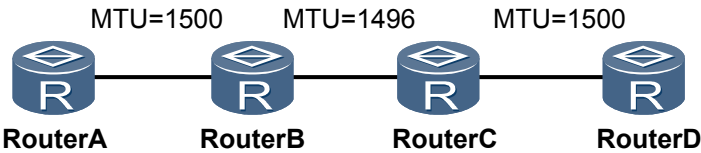
图 8-3 路径 MTU 自动发现组网示例图
