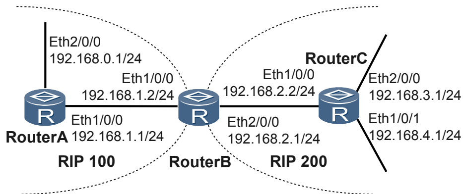
图 3-2 配置 RIP 引入外部路由组网图
