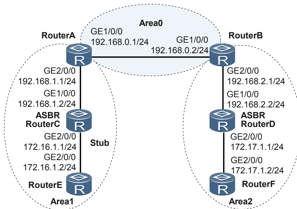
图 5-5 配置 OSPF 基本功能组网图
