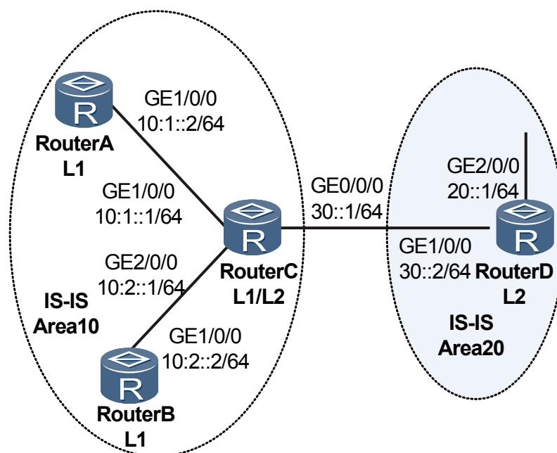
图 7-7 配置 IS-IS 的 IPv6 特性基本功能组网图
