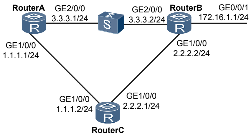
图 7-12 配置动态 BFD for IS-IS 组网图
