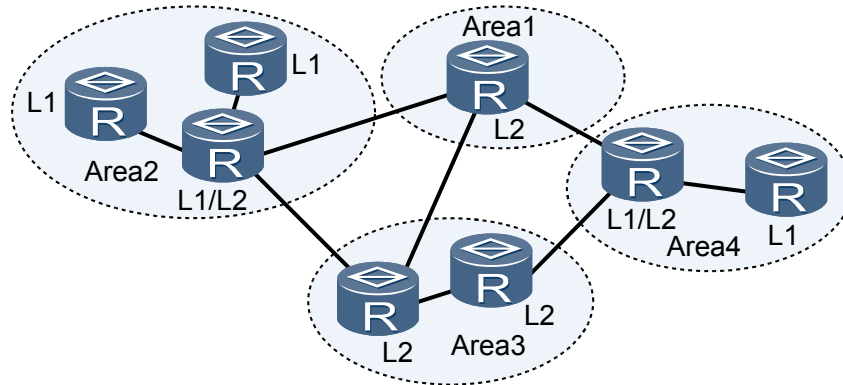
图 7-2 IS-IS 拓扑结构图之二
