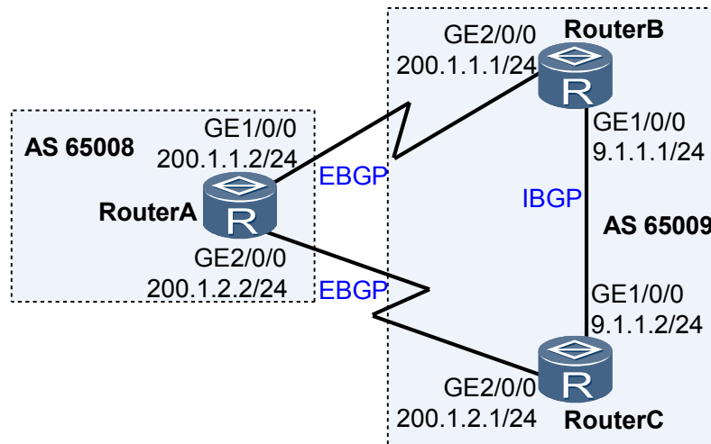
图 8-8 配置 BGP 的 MED 属性控制路由选择组网图
