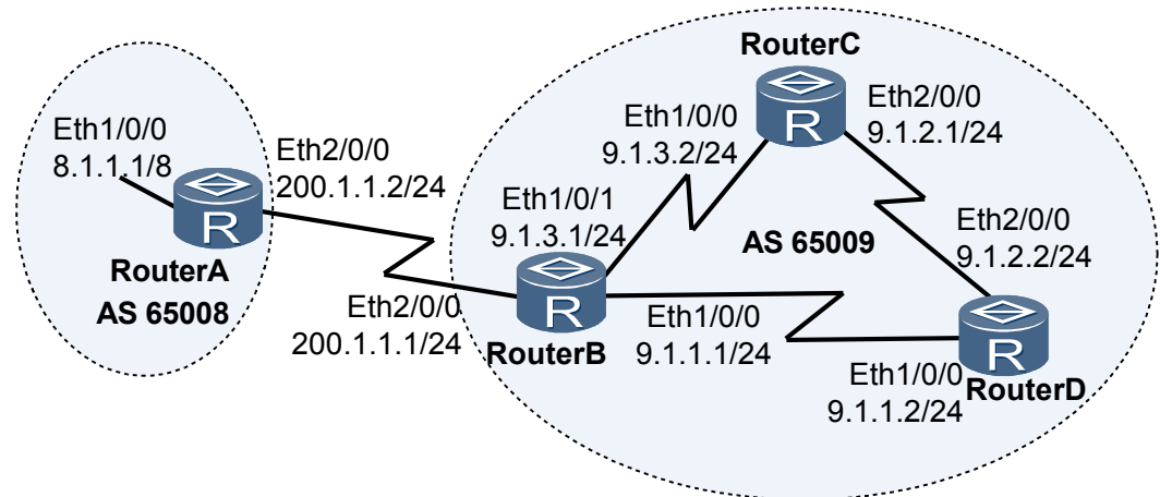
图 8-5 配置 BGP 基本组网图
