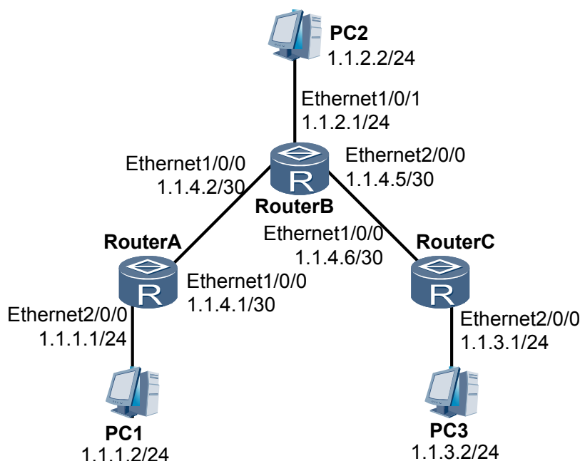
图 2-1 配置 IPv4 静态路由组网图
