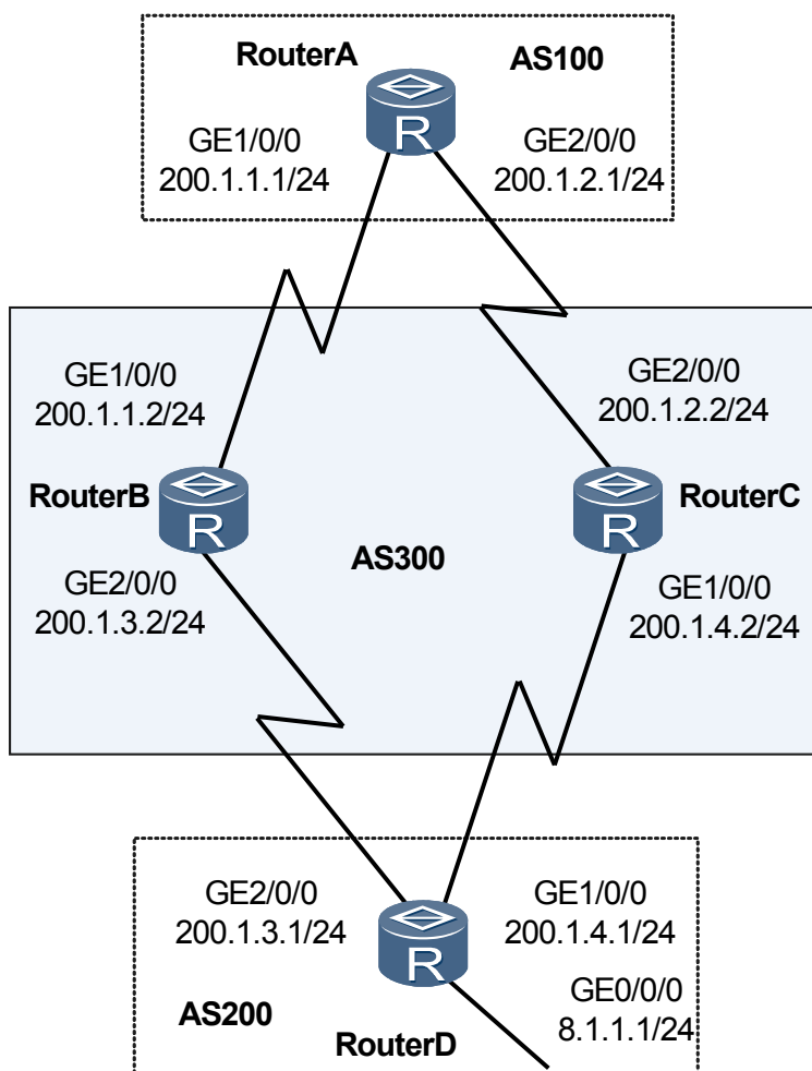
图 8-13 配置 BGP 负载分担组网图
