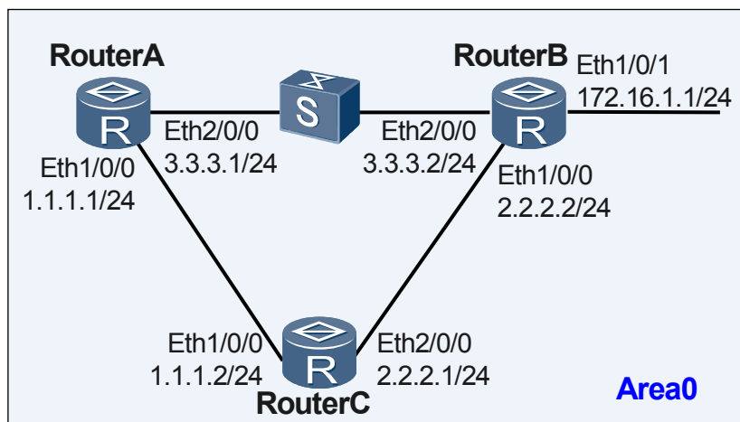
图 5-11 配置 BFD for OSPF 特性组网图
