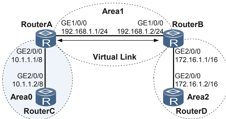
图 5-6 配置 OSPF 虚连接的组网图
