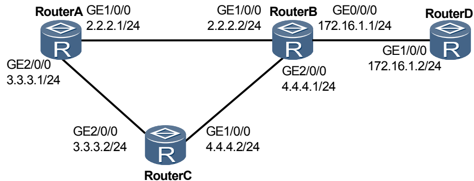
图 3-4 配置 BFD for RIP 组网图
