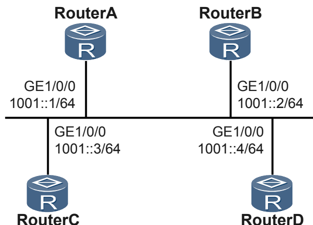
图 6-2 配置 OSPFv3 的 DR 选择组网图
