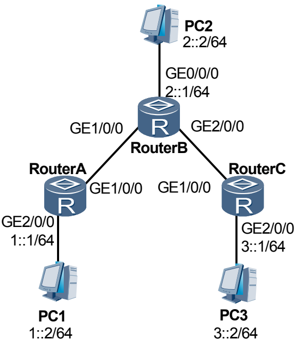
图 2-2 配置 IPv6 静态路由组网图
