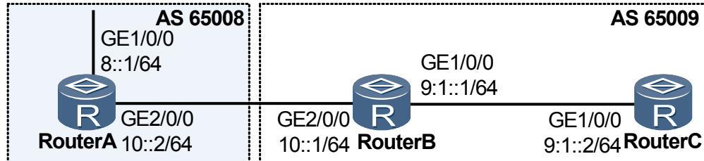
图 9-1 配置 BGP4+ 基本组网图
