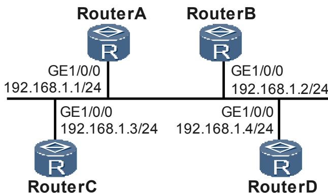
图 5-7 配置 OSPF 的 DR 选择组网图
