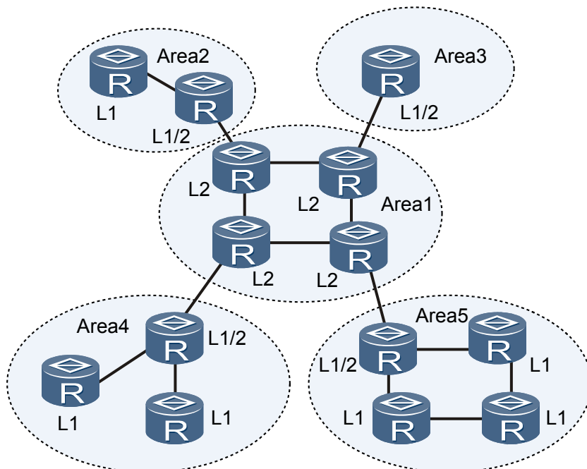
图 7-1 IS-IS 拓扑结构图之一
