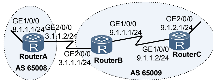
图 8-6 配置 BGP 与 IGP 交互配置组网图
