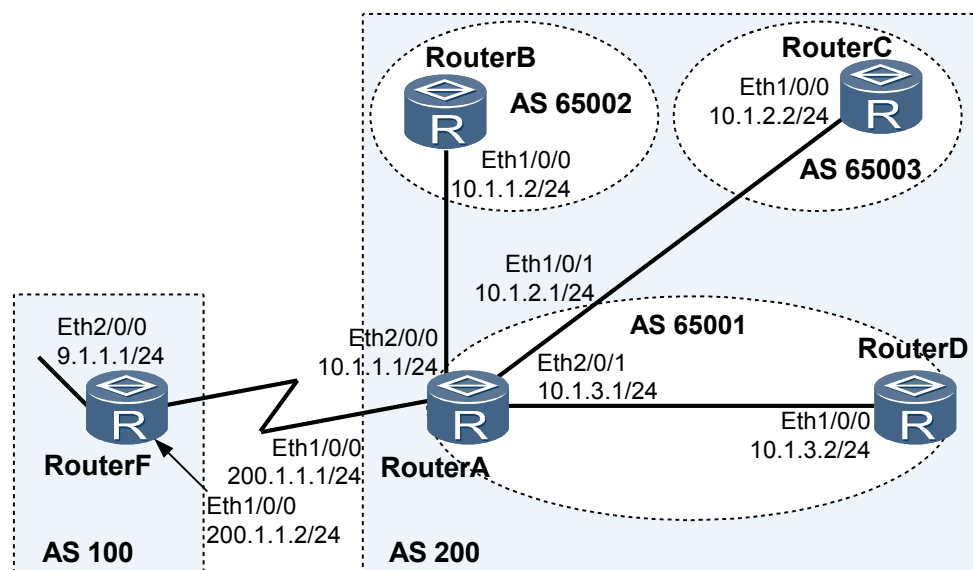
图 8-10 配置联盟组网图
