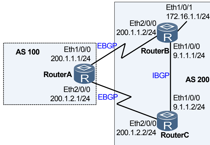
图 8-14 配置 BFD for BGP 组网图
