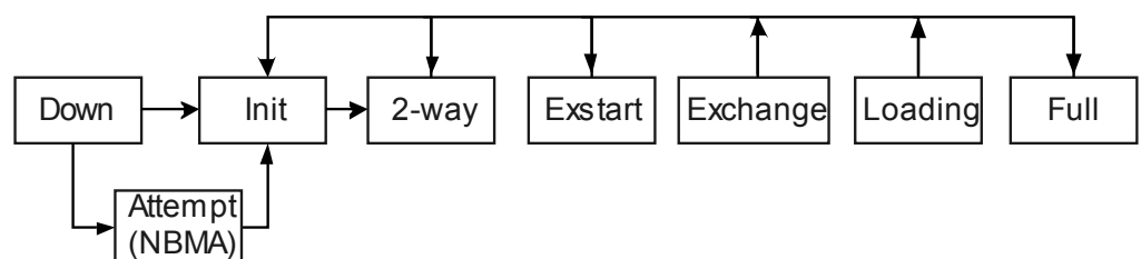
图 5-3 邻居状态机的变化
