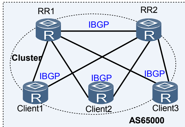
图 8-1 路由反射器集群
