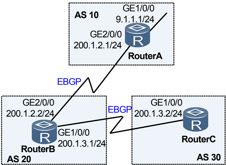
图 8-11 配置 BGP 团体组网图
