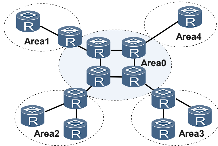
图 5-1 OSPF 区域划分
