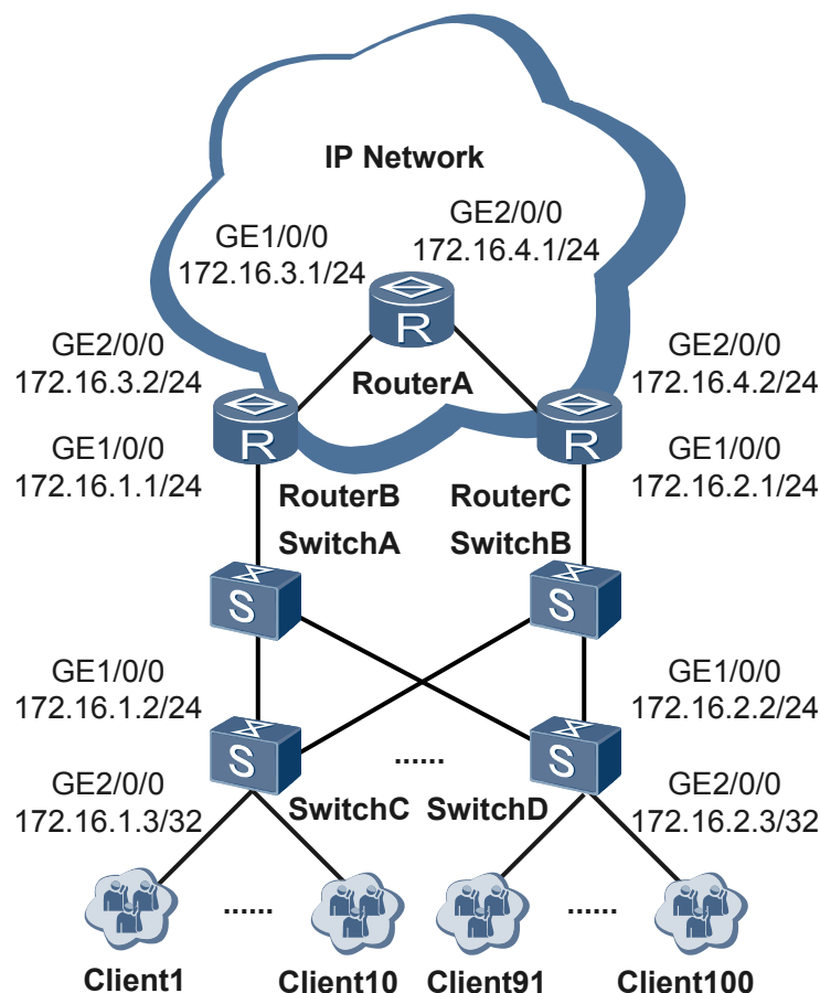
图 2-4 配置静态路由与 NQA 联动组网图
