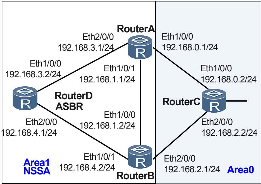
图 5-9 配置 OSPF NSSA 区域组网图
