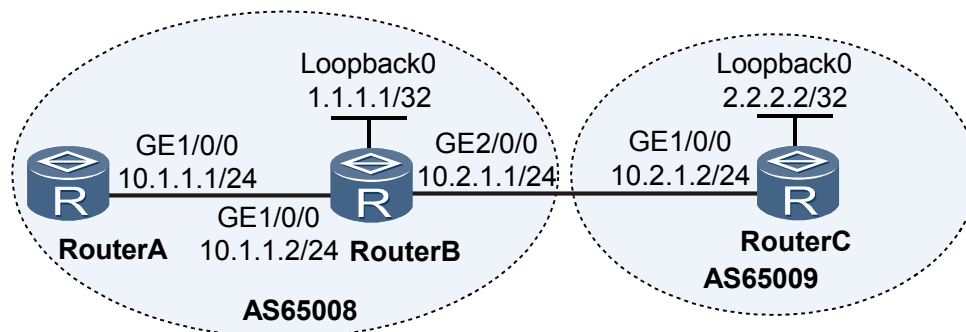
图 7-6 配置 IS-IS 和 BGP 交互组网图
