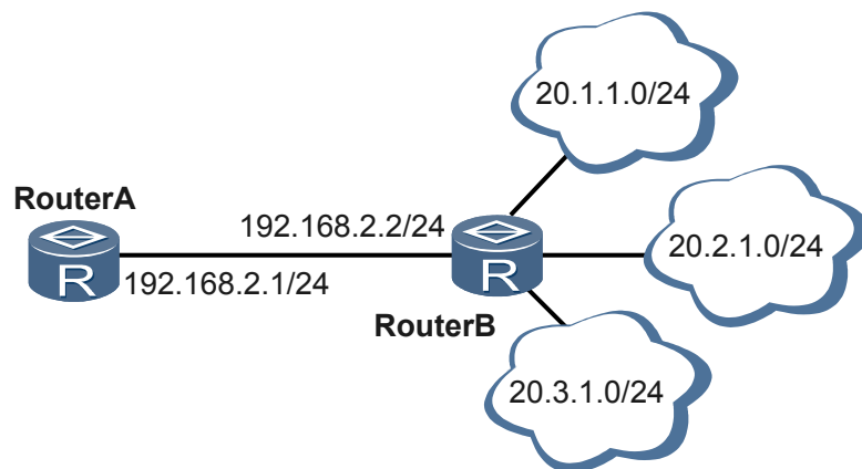
图 8-2 向对等体发送缺省路由典型组网图
