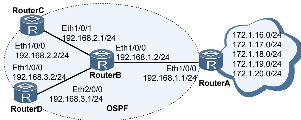
图 10-1 配置对接收和发布的路由过滤组网图
