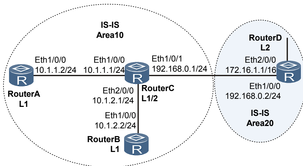
图 7-3 配置 IS-IS 基本功能组网图
