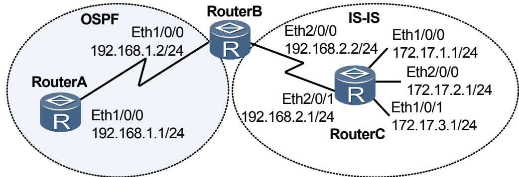
图 10-2 配置在路由引入时应用路由策略组网图
