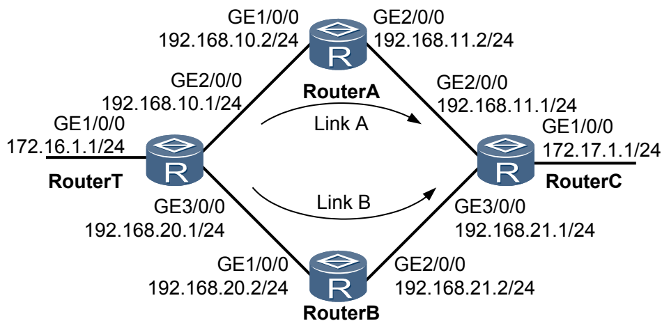
图 1-1 配置公网 IP FRR 功能组网图
