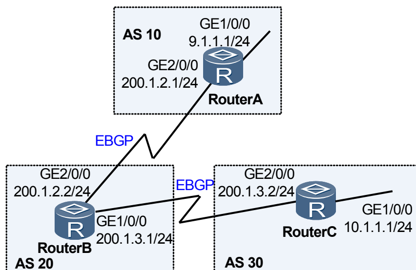
图 8-7 配置 AS_Path 过滤器组网图
