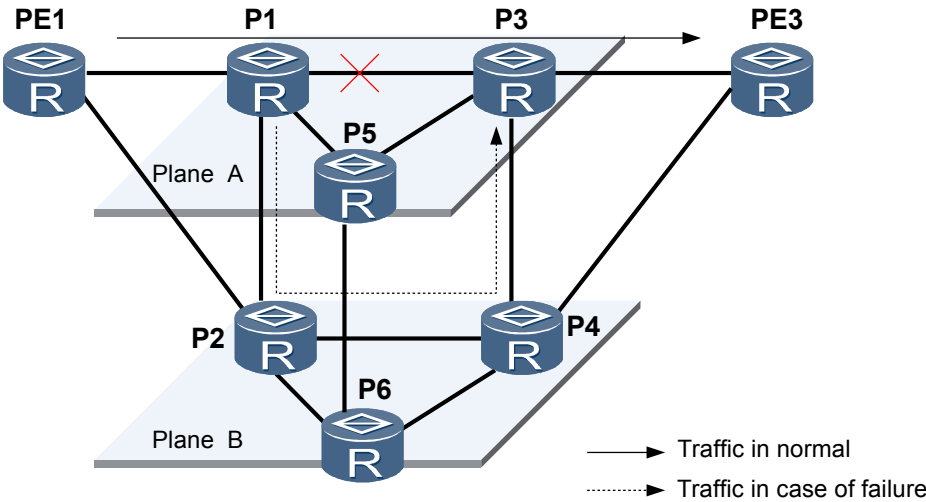
图 7-10 IS-IS Auto FRR 配置组网图
