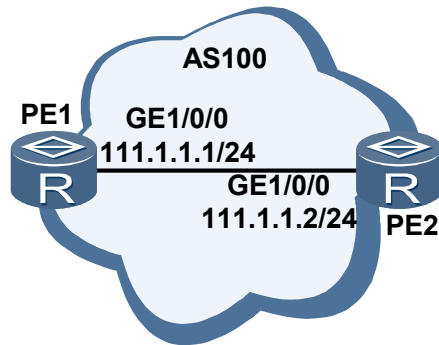
图 8-12 配置基于前缀的 BGP ORF 基本组网图
