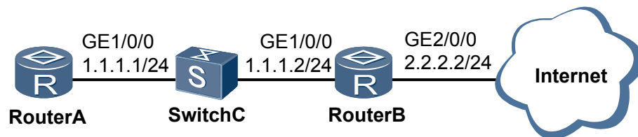
图 2-3 配置 BFD for IPv4 静态路由组网图
