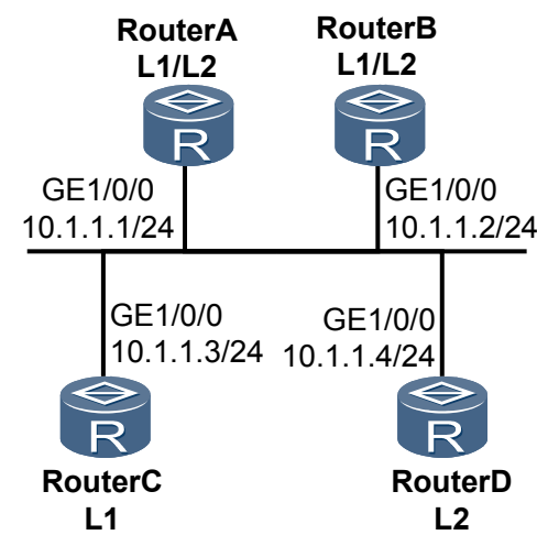
图 7-5 配置 IS-IS 的 DIS 选择组网图
