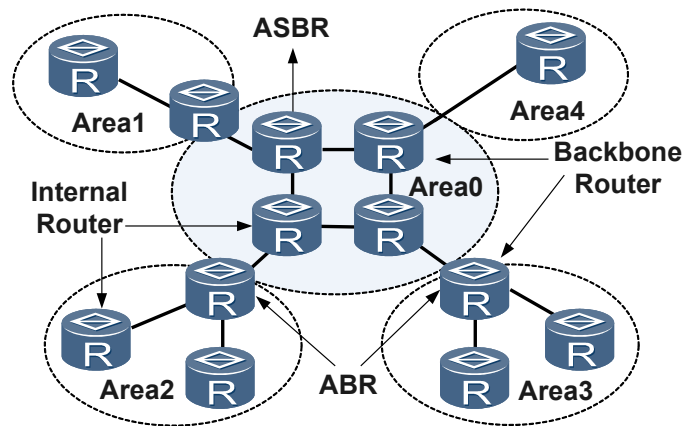
图 5-2 OSPF 路由器的类型
