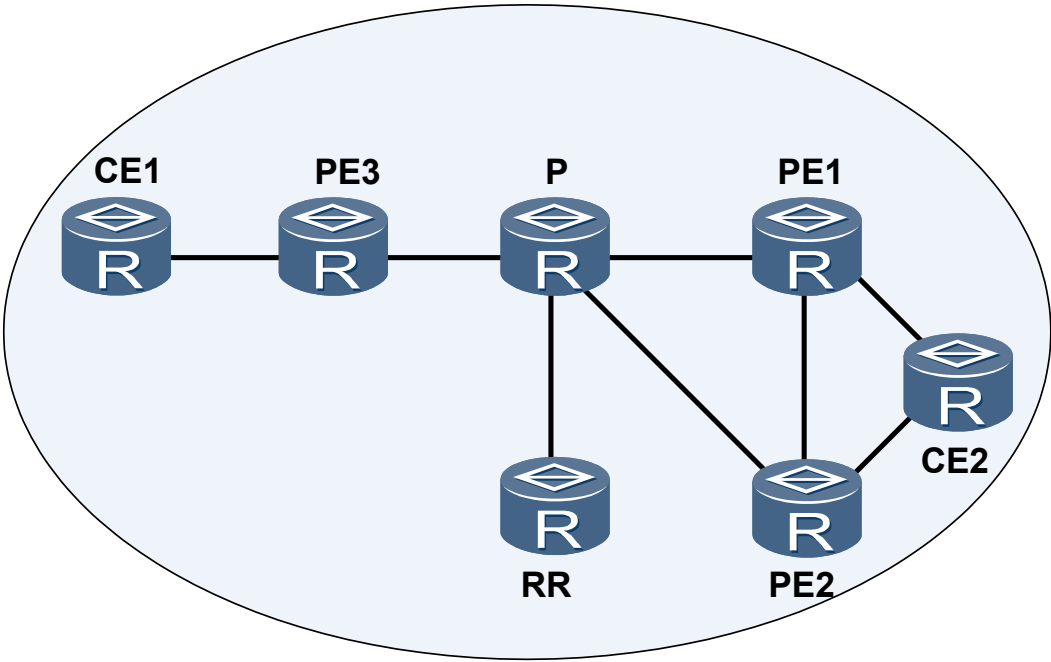
图 8-4 BGP 下一跳延时响应组网图
