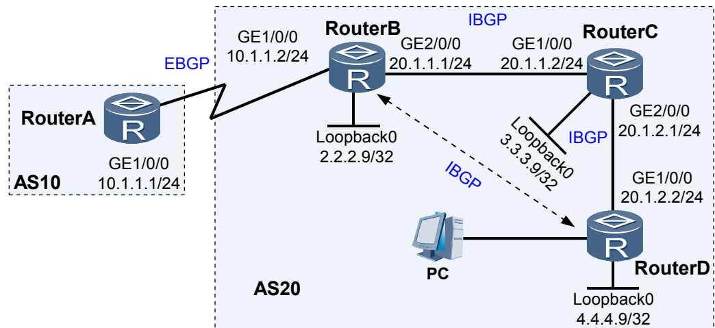
图 8-15 配置 BGP GTSM 特性组网图
