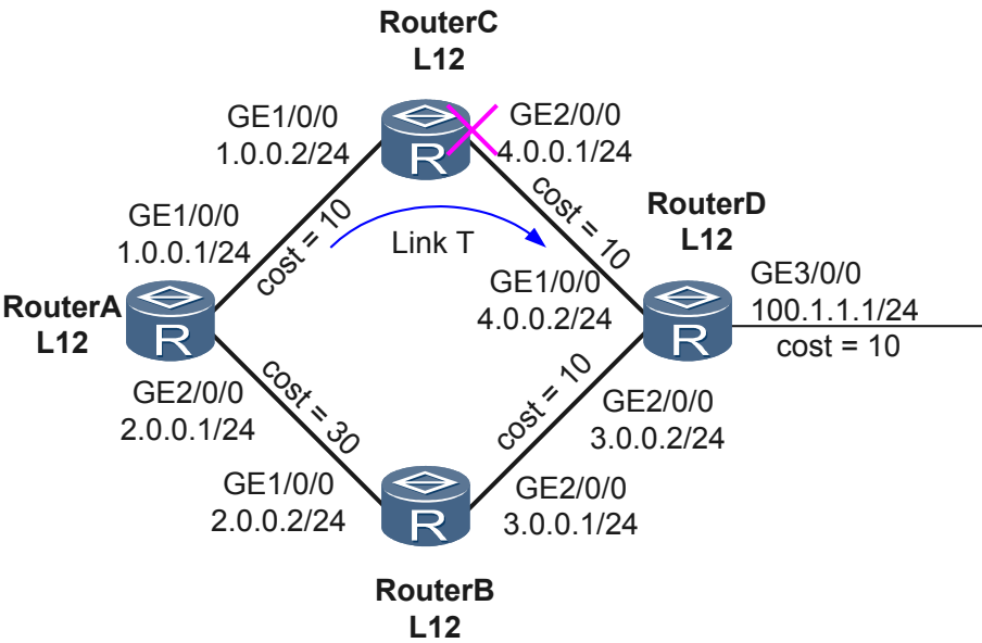
图 7-9 配置 IS-IS Auto FRR 组网图
