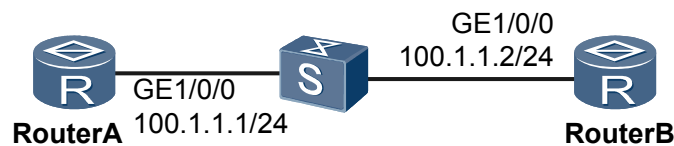
图 7-8 配置 IS-IS 快速收敛组网图
