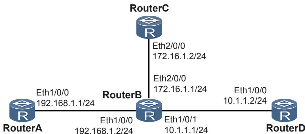
图 3-1 配置 RIP 版本组网图
