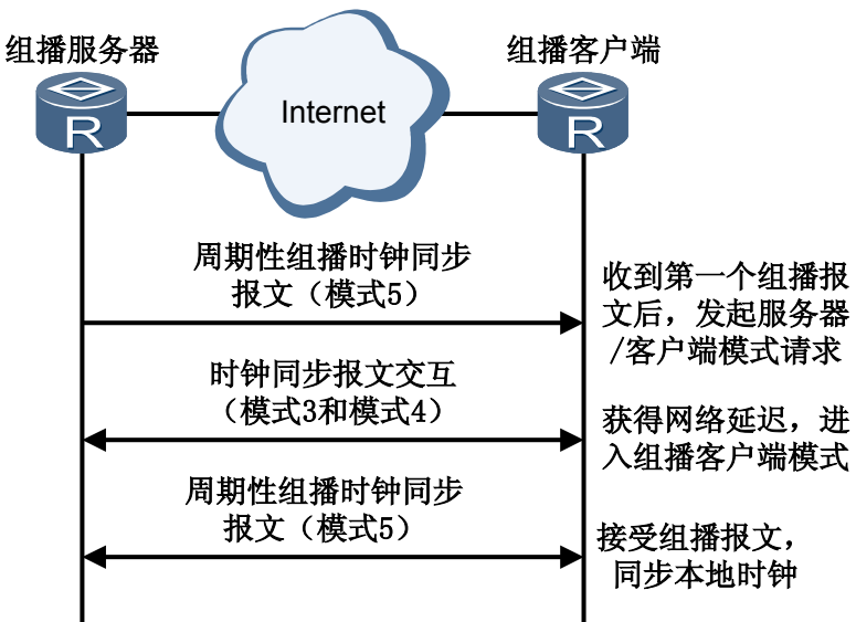
图 5-6 组播模式
