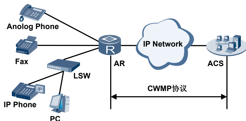
图 4-3 ACS 通过 CWMP 管理 AR1200
