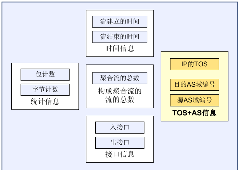
图 7-28 根据 TOS + AS 域进行聚合示意图
