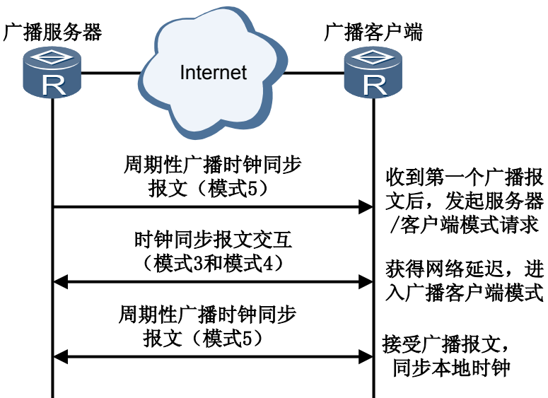
图 5-5 广播模式
