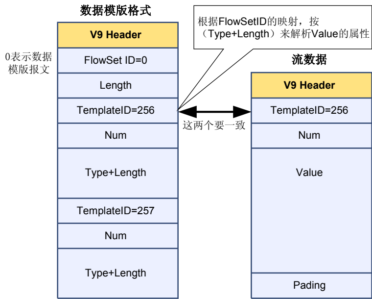
图 7-38 版本 9 流数据模板与流数据
