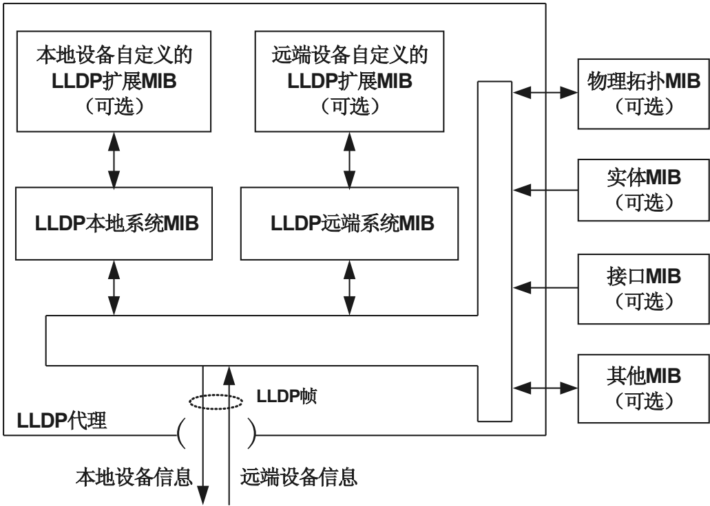
图 3-4 LLDP 结构框图
