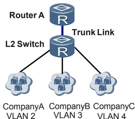
图 3-15 多个 VLAN 属于同一个三层设备互通组网图
