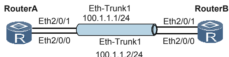
图 1-12 Eth-Trunk 组网图
