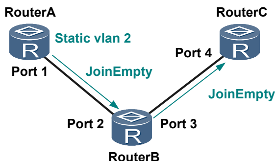
图 4-5 VLAN 属性的单向注册
