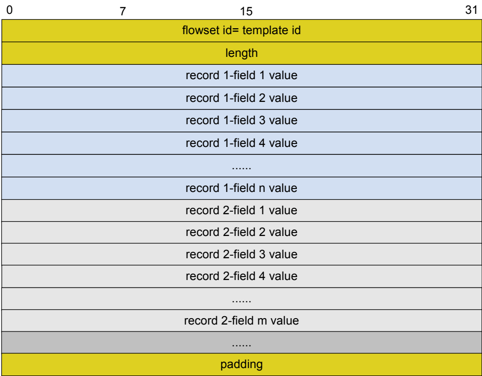
图 7-37 Data FlowSet 的报文格式
