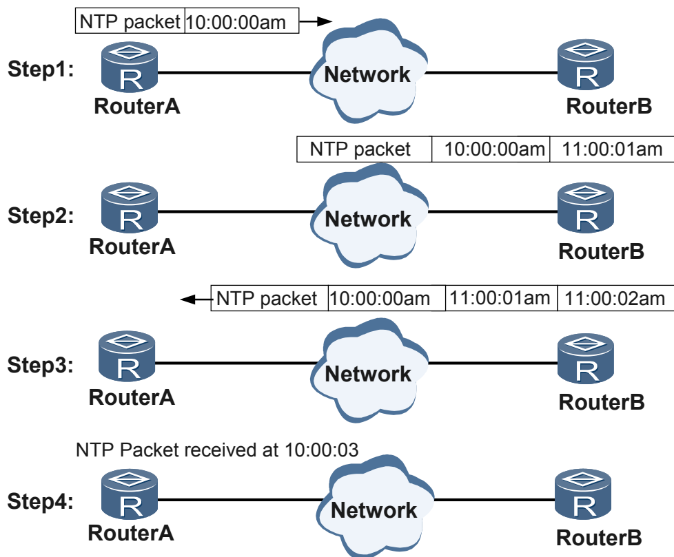
图 5-7 NTP 实现过程图
