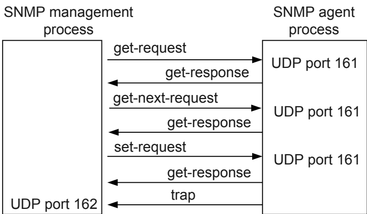
图 1-4 SNMP 的报文操作
