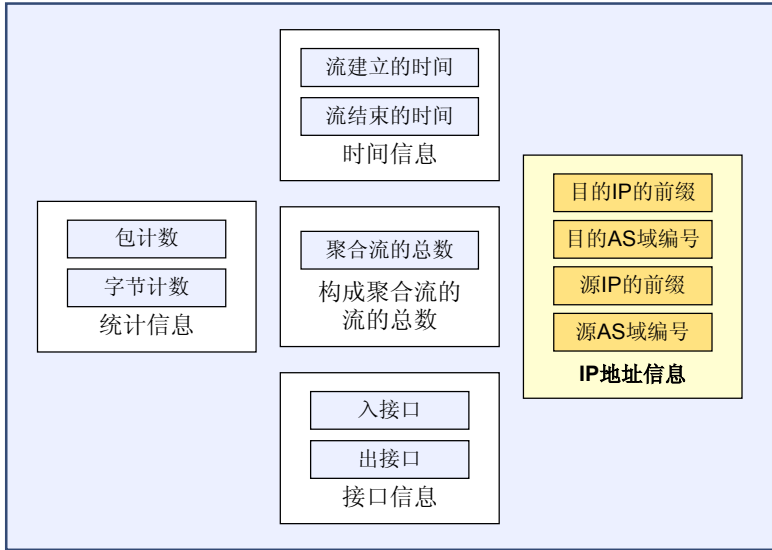
图 7-27 根据源 IP 地址的前缀和目的 IP 地址的前缀进行聚合示意图
