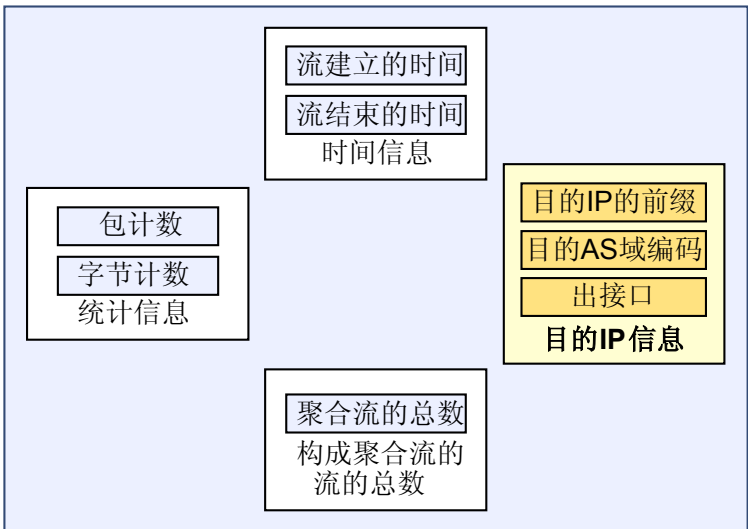
图 7-6 根据目的 IP 地址的前缀聚合示意图
