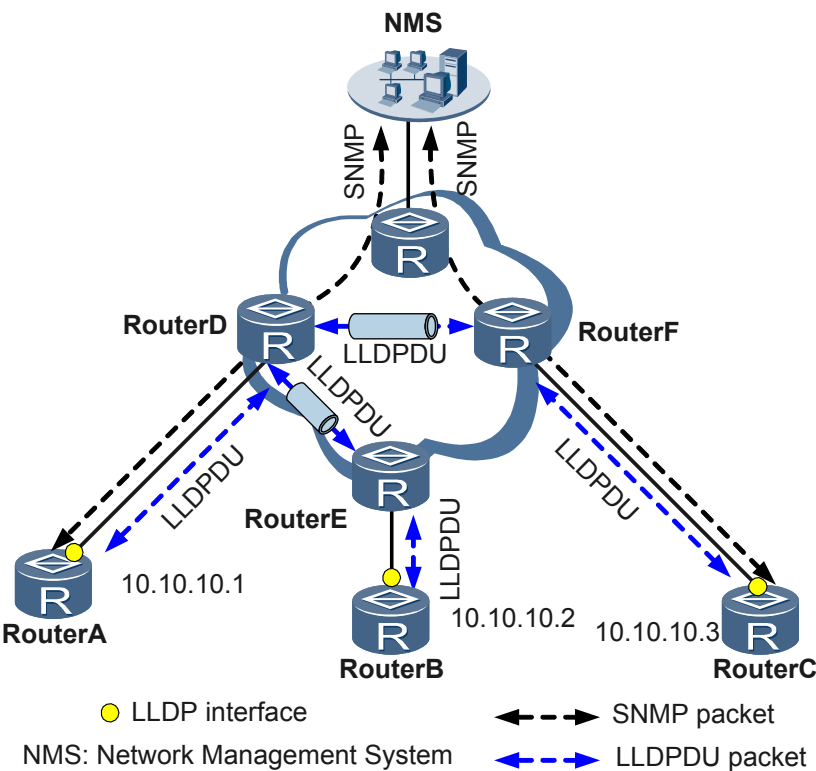
图 3-6 多邻居组网方式
