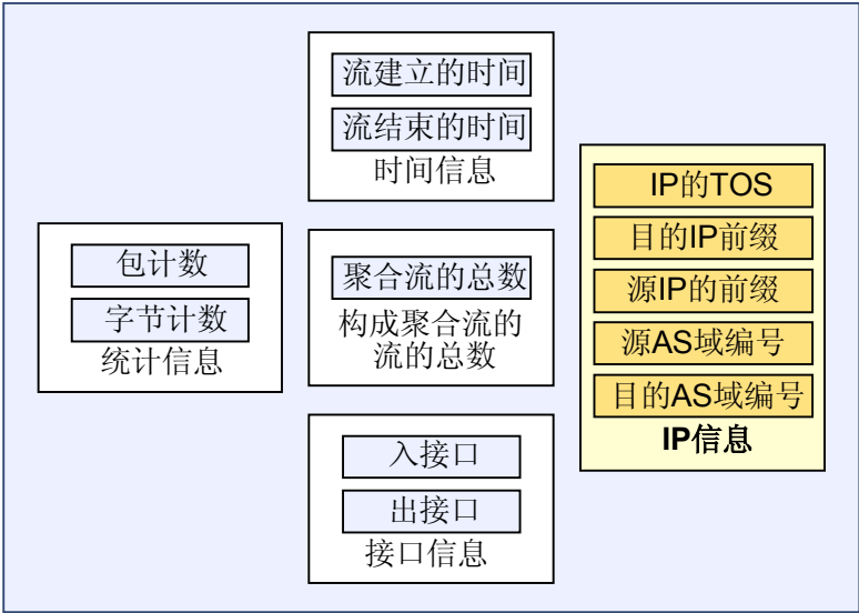
图 7-13 根据 TOS + IP 地址前缀进行聚合示意图
