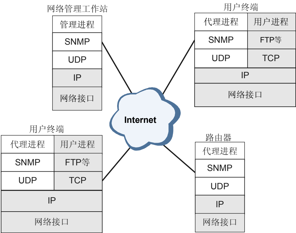
图 1-1 SNMP 典型配置
