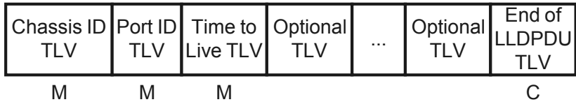
图 3-2 LLDPDU 结构图
