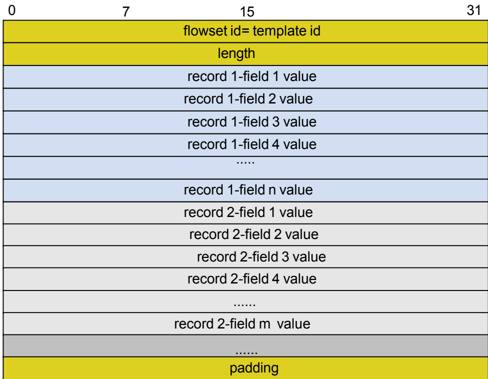
图 7-16 Data FlowSet 的报文格式
