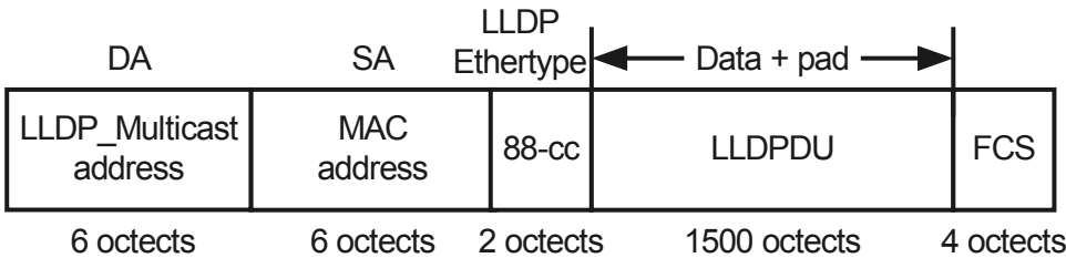
图 3-1 LLDP 报文结构
