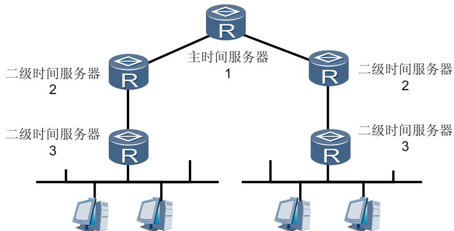
图 5-1 NTP 网络结构
