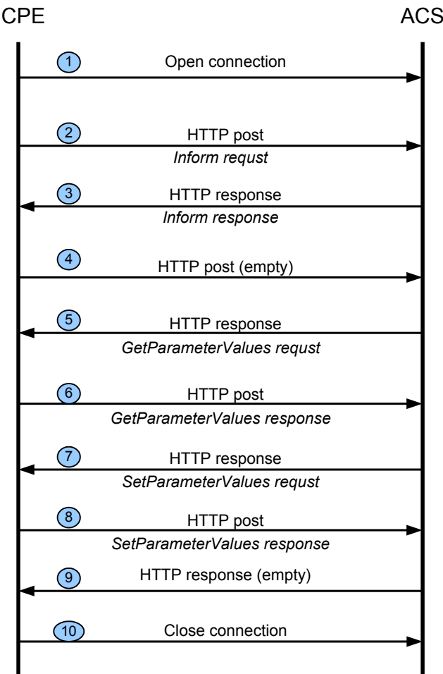
图 4-2 CWMP 消息交互示例
