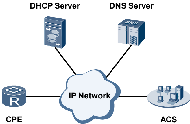
图 4-1 CWMP 端到端框架模型图
