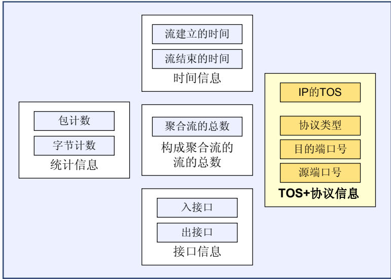
图 7-29 根据 TOS + 协议类型进行聚合示意图
