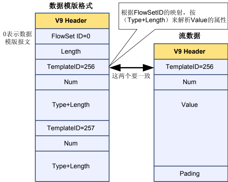
图 7-38 版本 9 流数据模板与流数据
