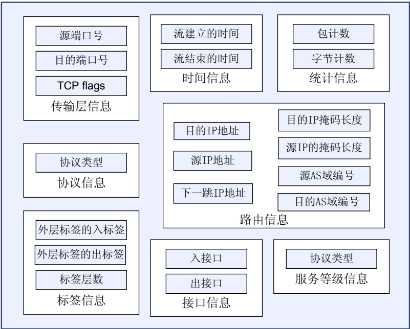
图 7-21 版本 5 信息
