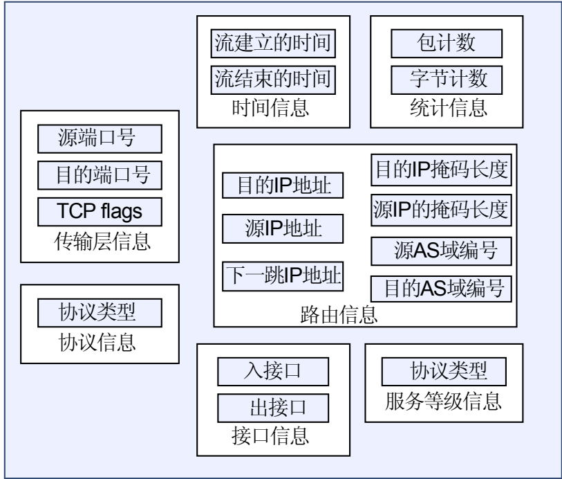
图 7-3 版本 5 信息
