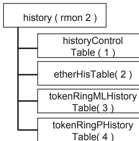
图 2-3 历史组
