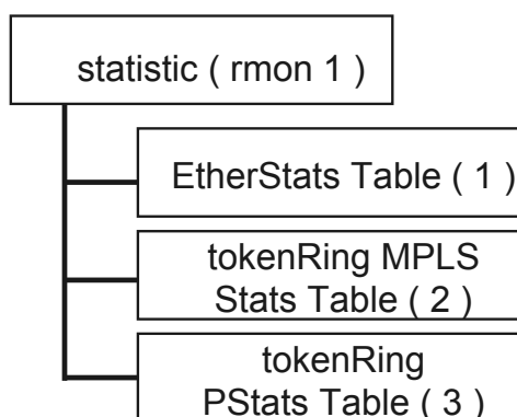
图 2-2 统计组
