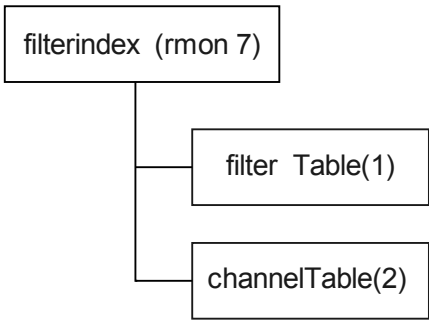
图 2-7 过滤组
