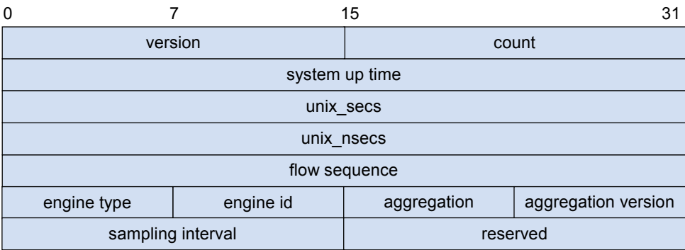
图 7-22 Netream v8 报文头
