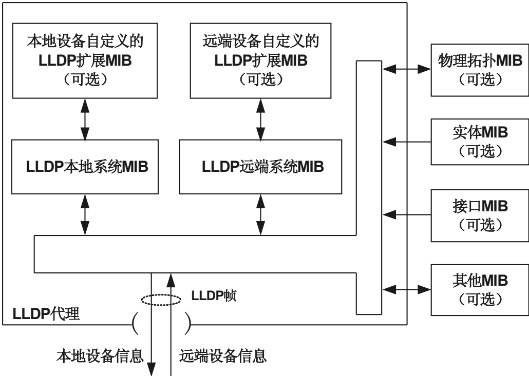
图 3-4 LLDP 结构框图
