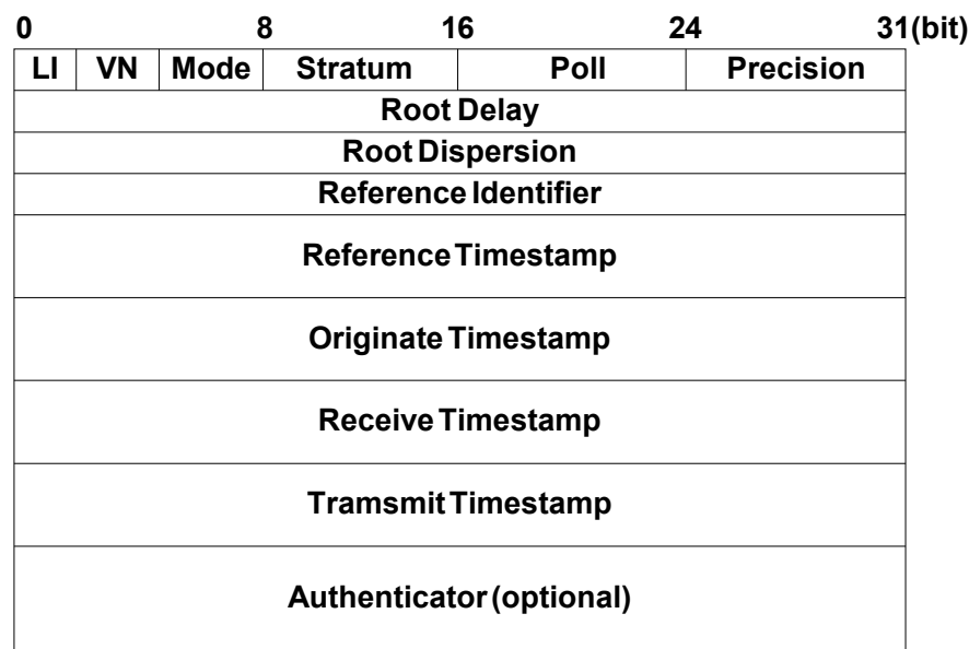
图 5-2 NTP 报文结构
