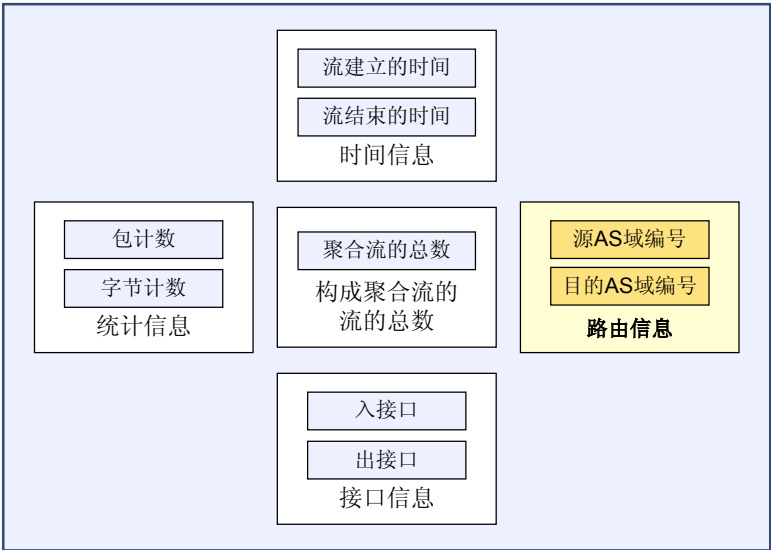
图 7-23 根据 AS 域进行聚合示意图
