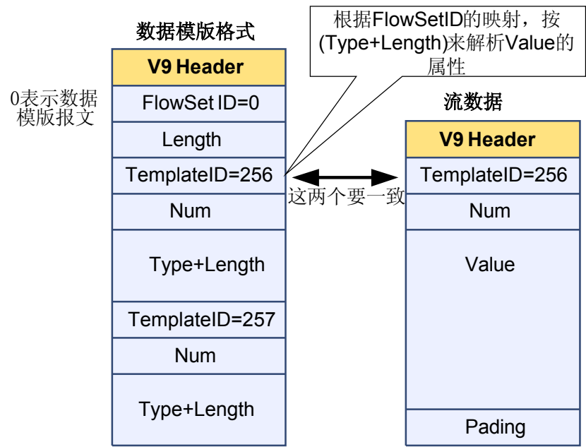
图 7-17 版本 9 流数据模板与流数据
