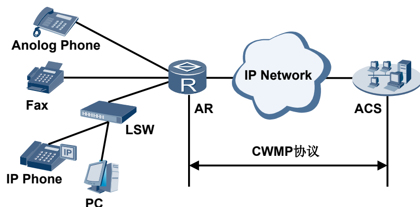
图 4-3 ACS 通过 CWMP 管理 AR200-S
