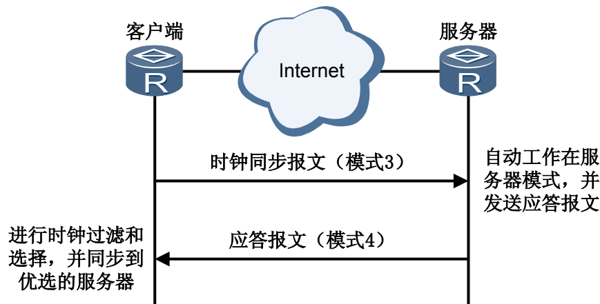
图 5-3 客户/服务器模式
