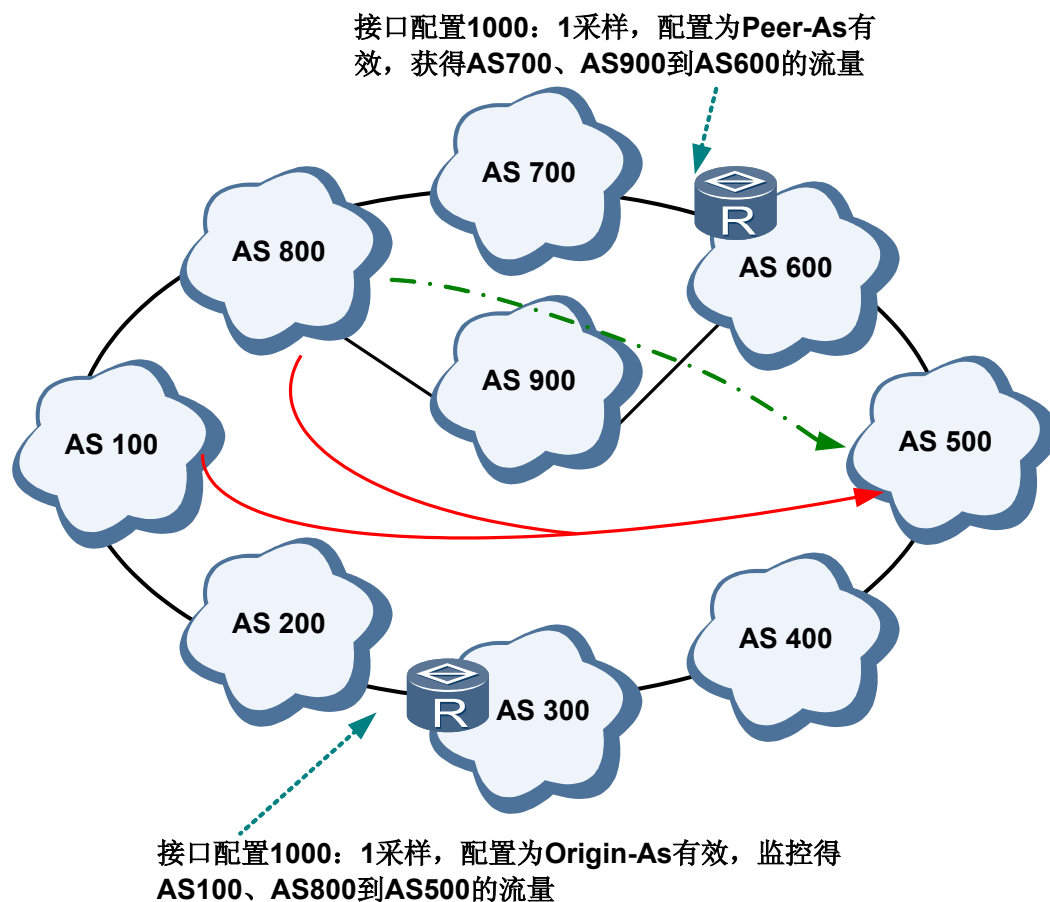
图 7-39 AS 域间规划示意图
