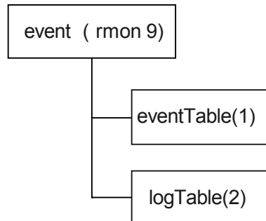
图 2-9 事件组
