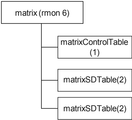
图 2-6 矩阵组
