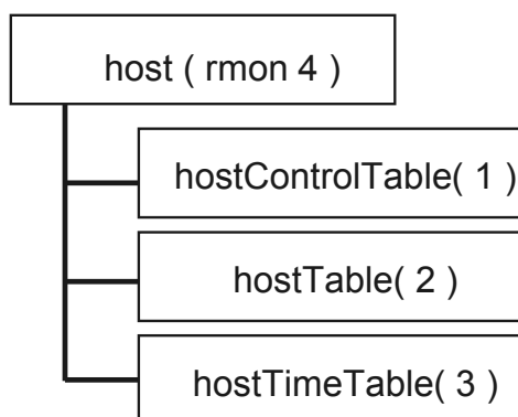
图 2-4 host 组
