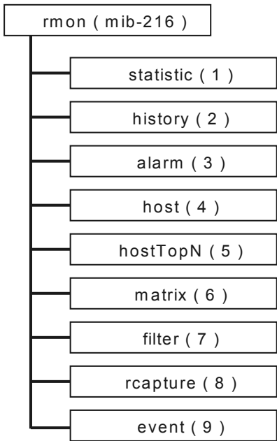
图 2-1 RMON MIB 组
