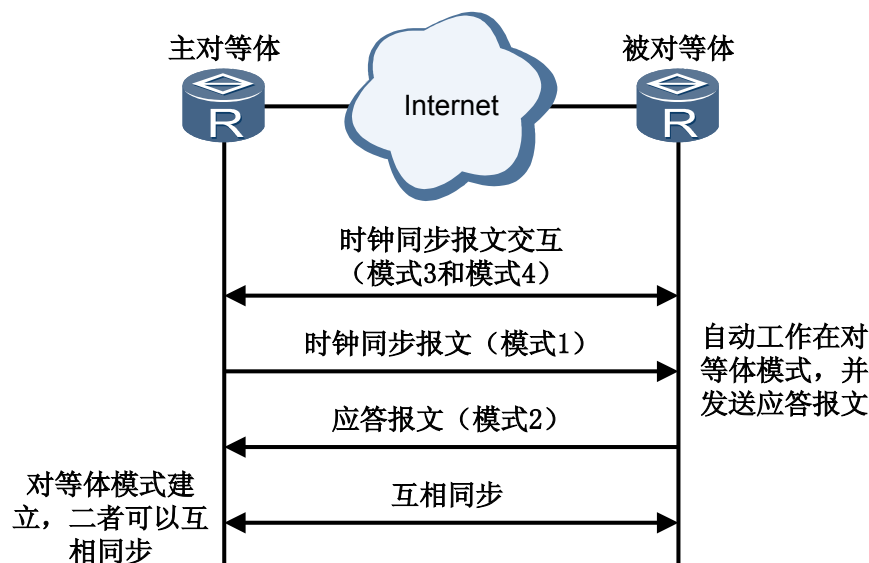
图 5-4 对等体模式
