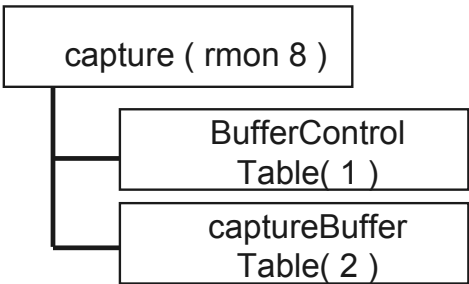
图 2-8 捕获组
