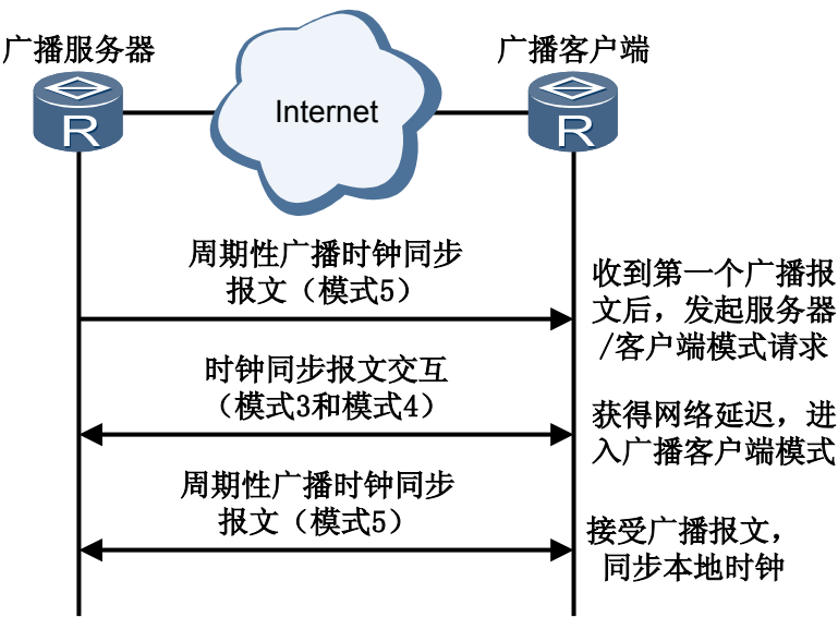
图 5-5 广播模式
