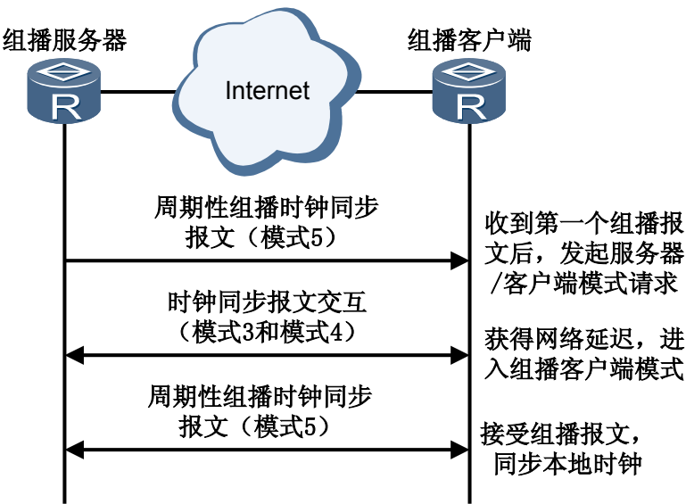
图 5-6 组播模式
