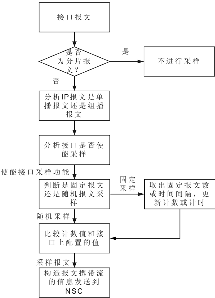
图 7-18 NetStream 采样处理流程
