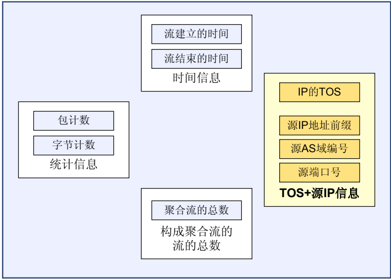
图 7-31 根据 TOS + 源 IP 地址前缀进行聚合示意图
