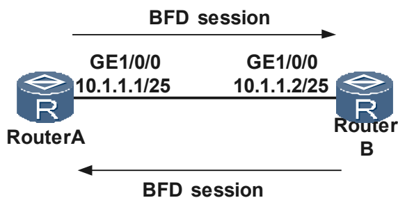
图 3-7 单跳 BFD for IP
