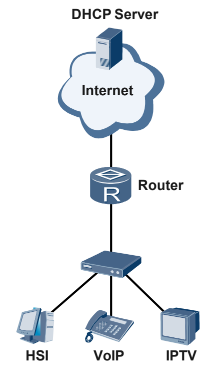
图 3-18 Voice VLAN 的应用组网图
