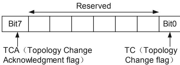
图 5-7 Flag 字段格式
