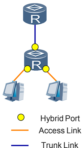
图 3-4 端口示意图
