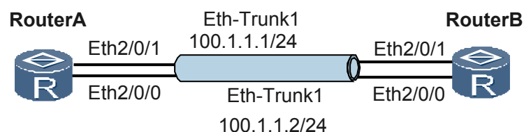
图 1-12 Eth-Trunk 组网图
