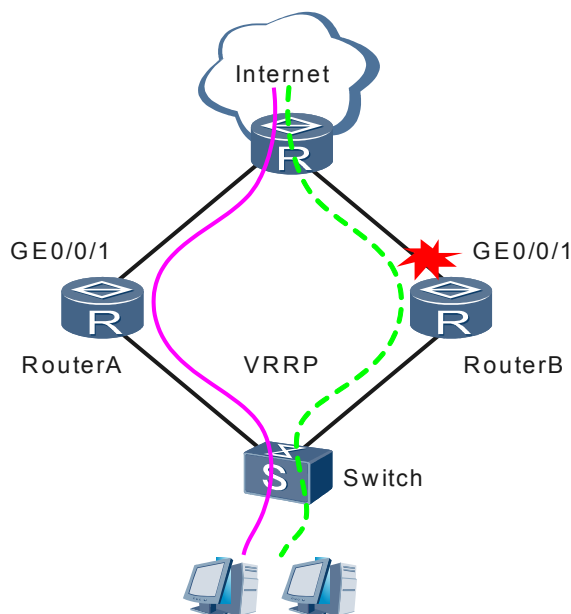
图 2-6 VRRP 监视接口的典型组网图
