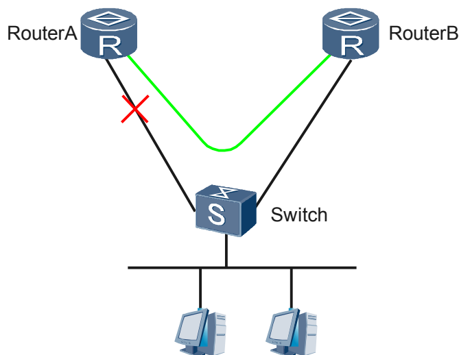
图 2-7 VRRP 快速切换组网图
