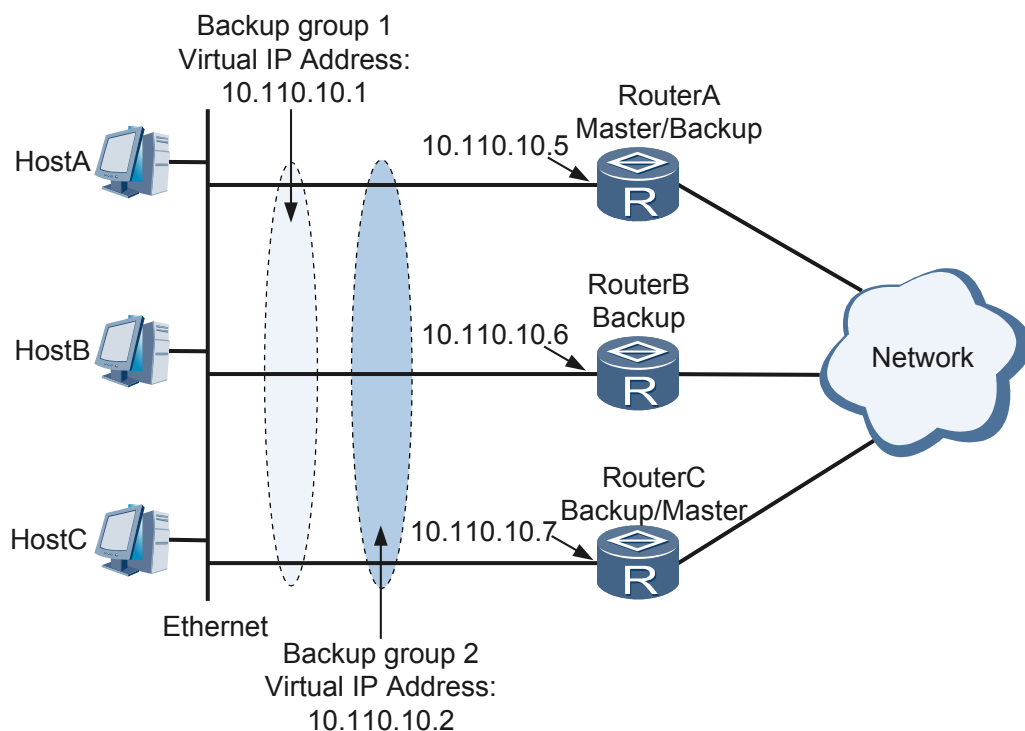
图 2-4 VRRP 负载分担示意图
