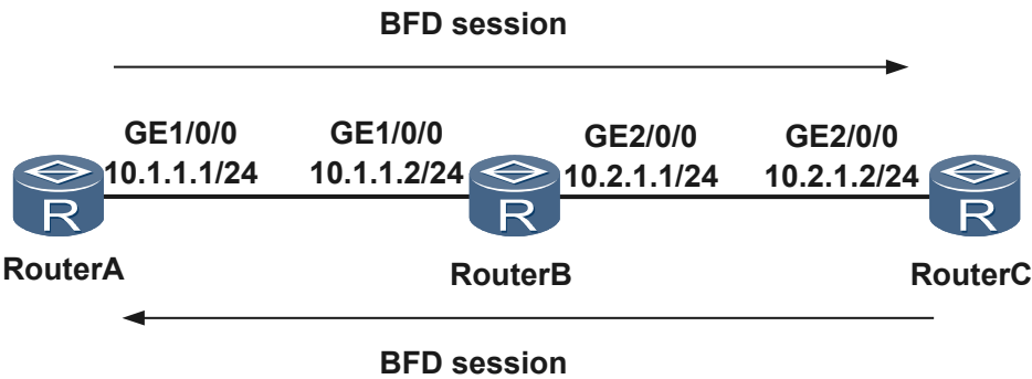
图 3-3 多跳 BFD for IP
