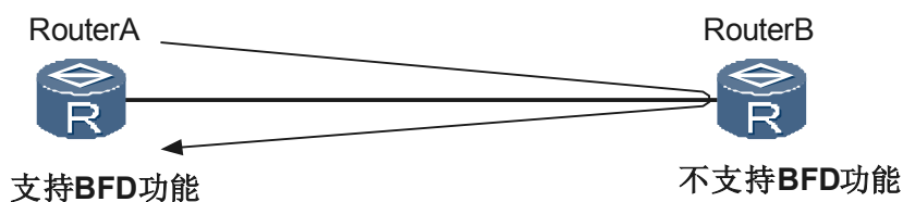
图 3-9 单臂 ECHO 功能组网示意图
