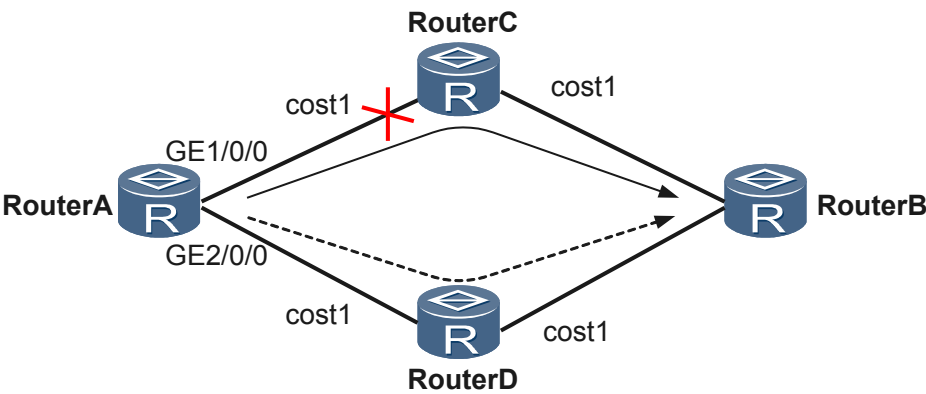
图 3-4 BFD for OSPF 组网图
