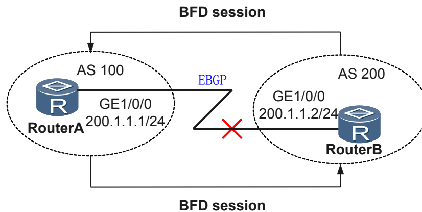
图 3-6 BFD for BGP 组网图
