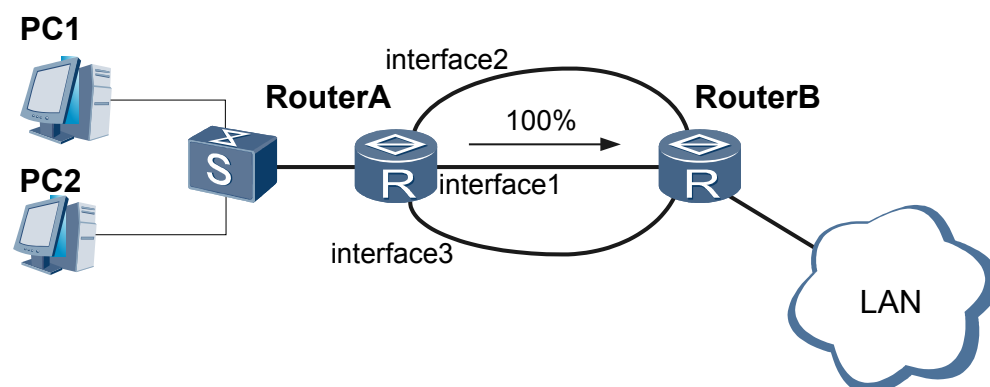
图 1-1 主备备份示意图
