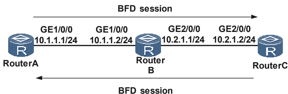
图 3-8 多跳 BFD for IP
