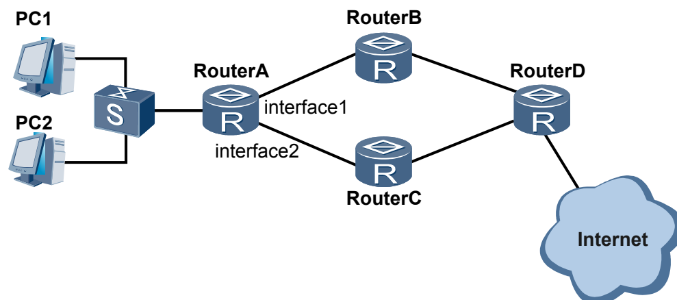
图 1-2 接口备份与 NQA 联动示意图
