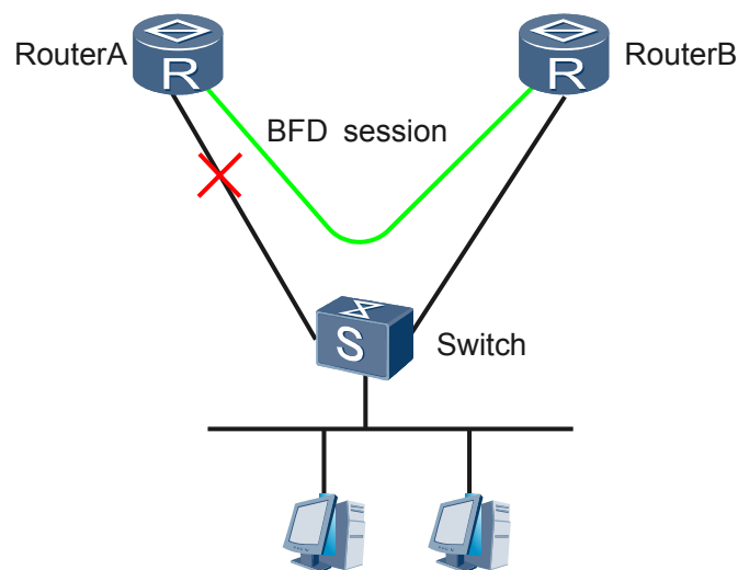
图 3-5 VRRP Track BFD 典型组网
