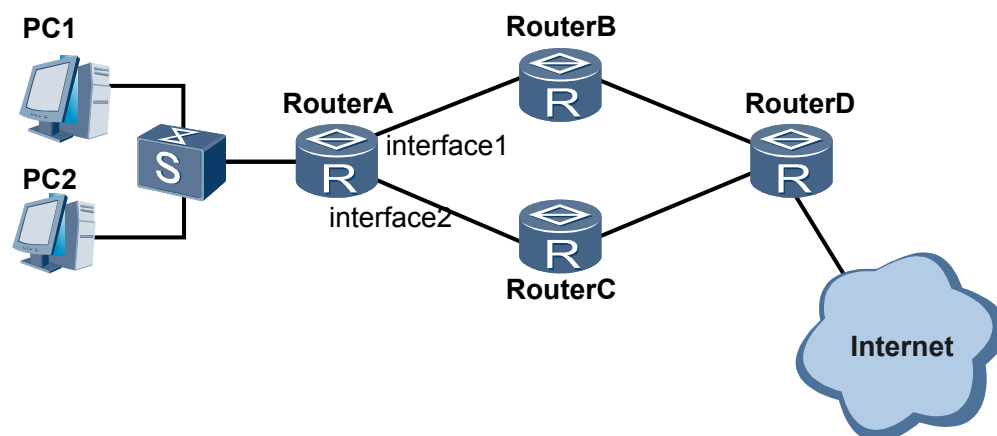
图 1-4 接口备份与路由联动示意图
