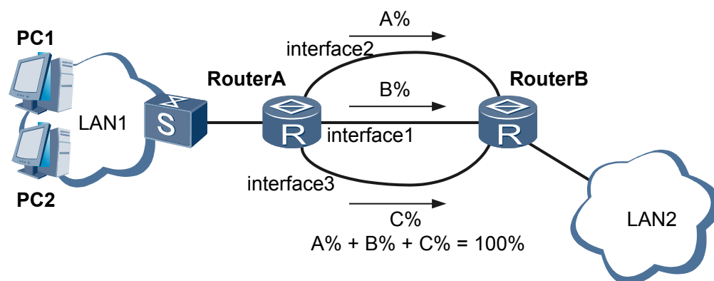
图 1-5 负载分担示意图
