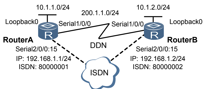
图 1-6 接口备份应用场景
