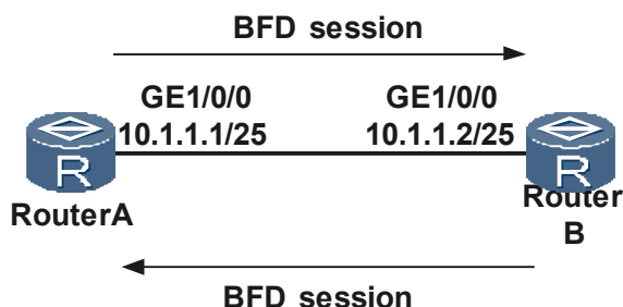
图 3-7 单跳 BFD for IP
