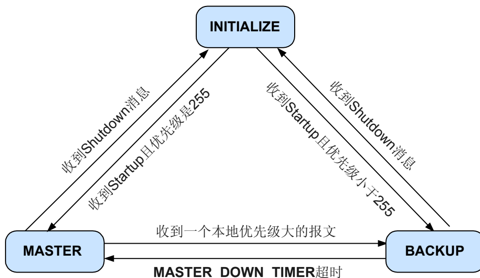
图 2-3 VRRP 状态机的转换
