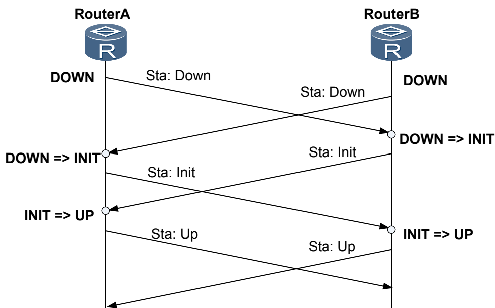
图 3-1 BFD 会话连接建立
