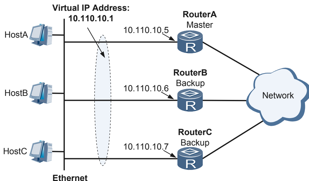
图 2-1 虚拟路由器示意图
