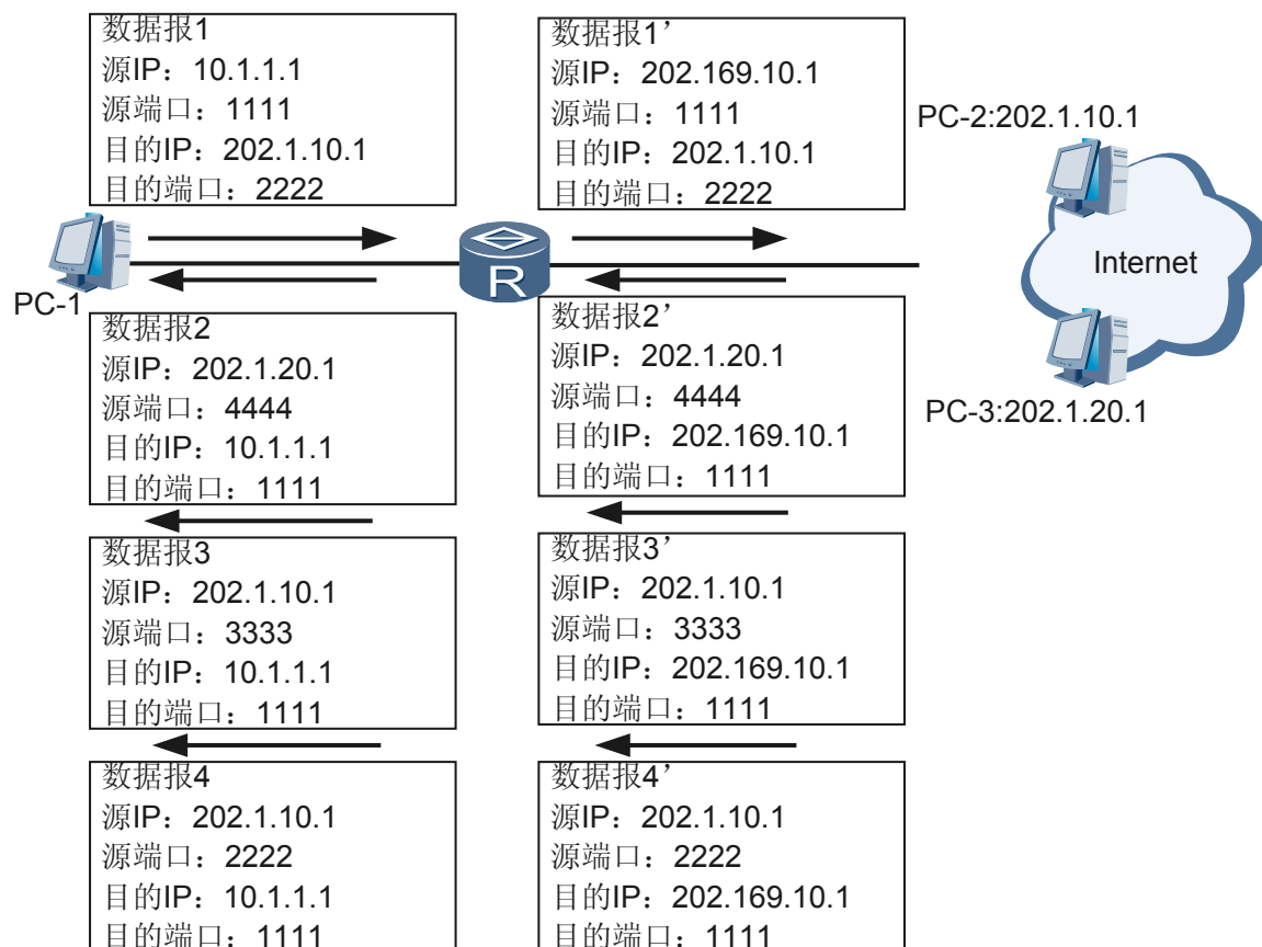
图 7-8 NAT 过滤应用
