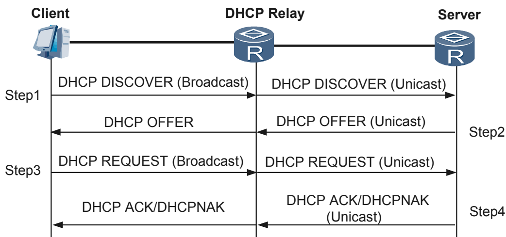
图 6-6 DHCP 客户端与 DHCP 服务器通过 DHCP 中继的交互过程
