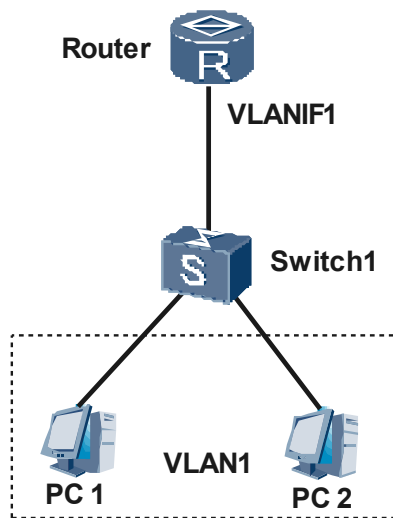
图 4-7 VLAN 内 ND 代理典型组网图
