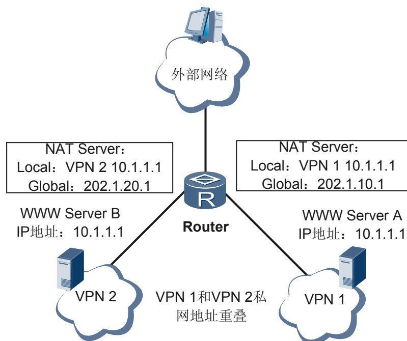
图 7-7 VPN 关联的 NAT Server
