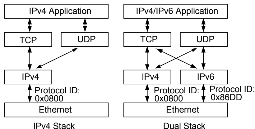
图 4-5 单协议栈与双协议栈结构（以太网）
