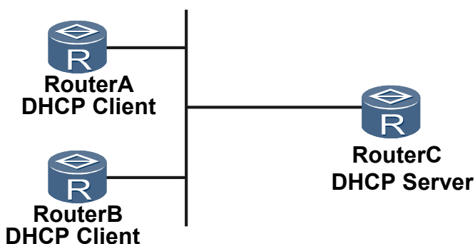
图 6-7 AR3200 接口作为 DHCP Client 的典型组网
