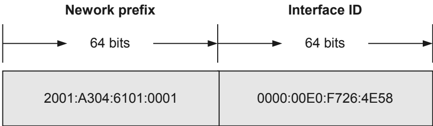
图 4-1 地址 2001:A304:6101:1:0000:E0:F726:4E58 /64 的构成示意图
