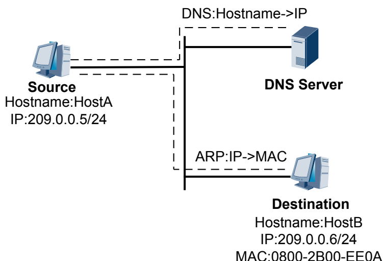
图 1-3 主机名、IP 地址和物理地址之间的关系
