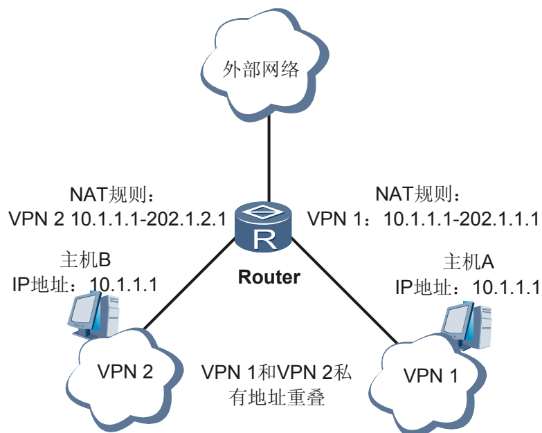
图 7-6 VPN 关联的源 NAT
