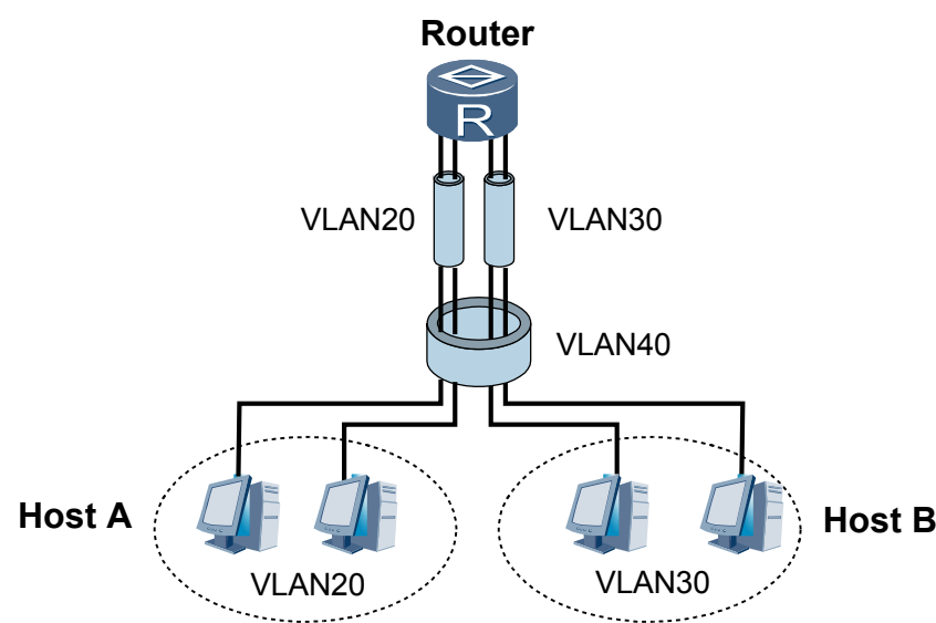
图 2-7 VLAN 间 Proxy ARP 典型组网图
