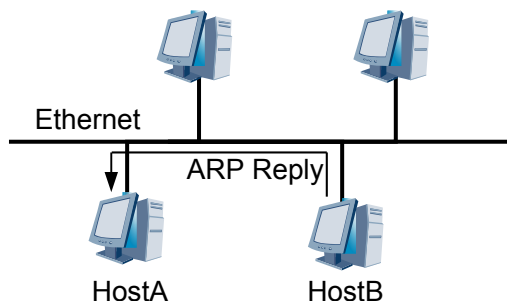
图 2-2 ARP 响应过程
