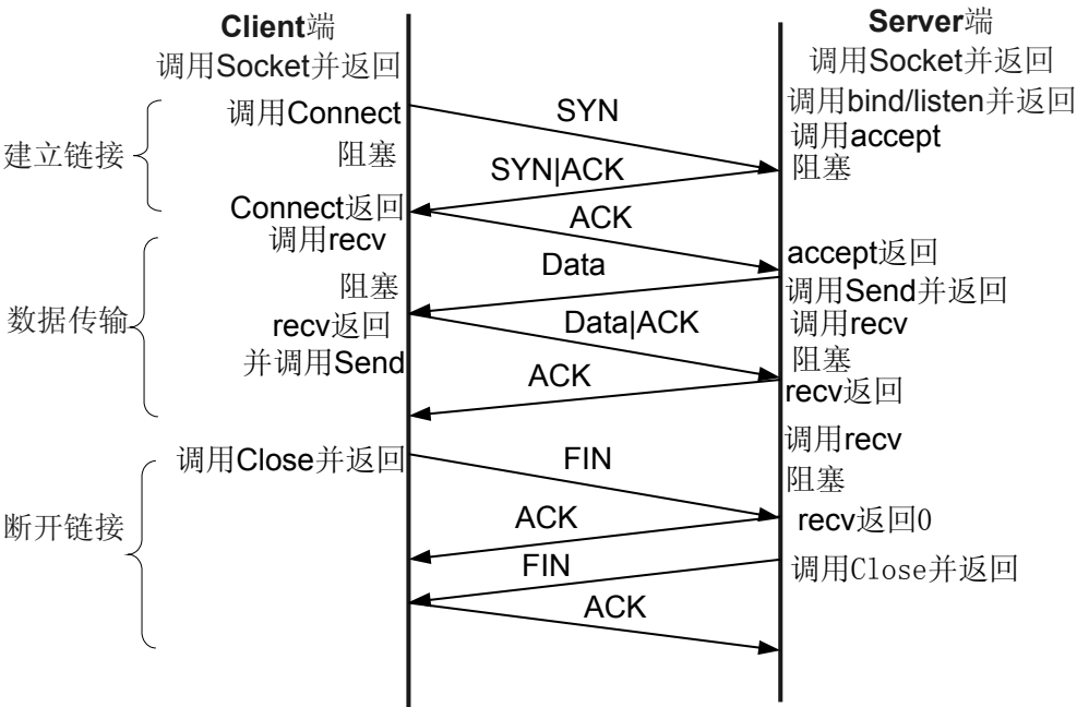
图 3-2 TCP 连接建立和拆除过程
