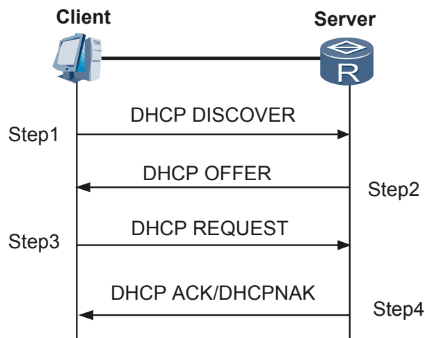
图 6-4 首次登录网络时 DHCP 客户端与 DHCP 服务器的交互过程
