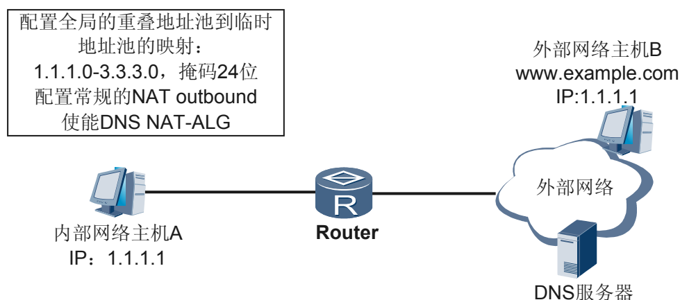
图 7-4 两次 NAT 示意图
