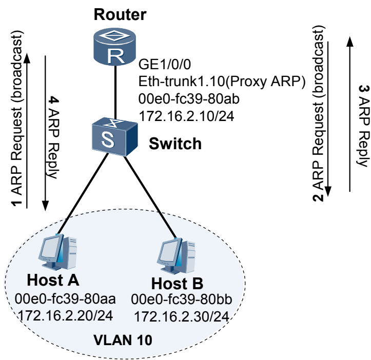
图 2-6 VLAN 内 Proxy ARP 典型组网图
