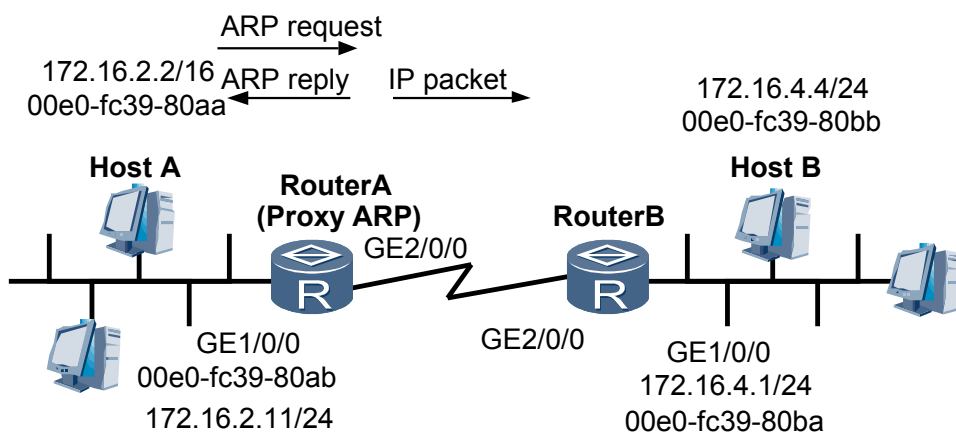
图 2-5 路由式 Proxy ARP 典型组网图
