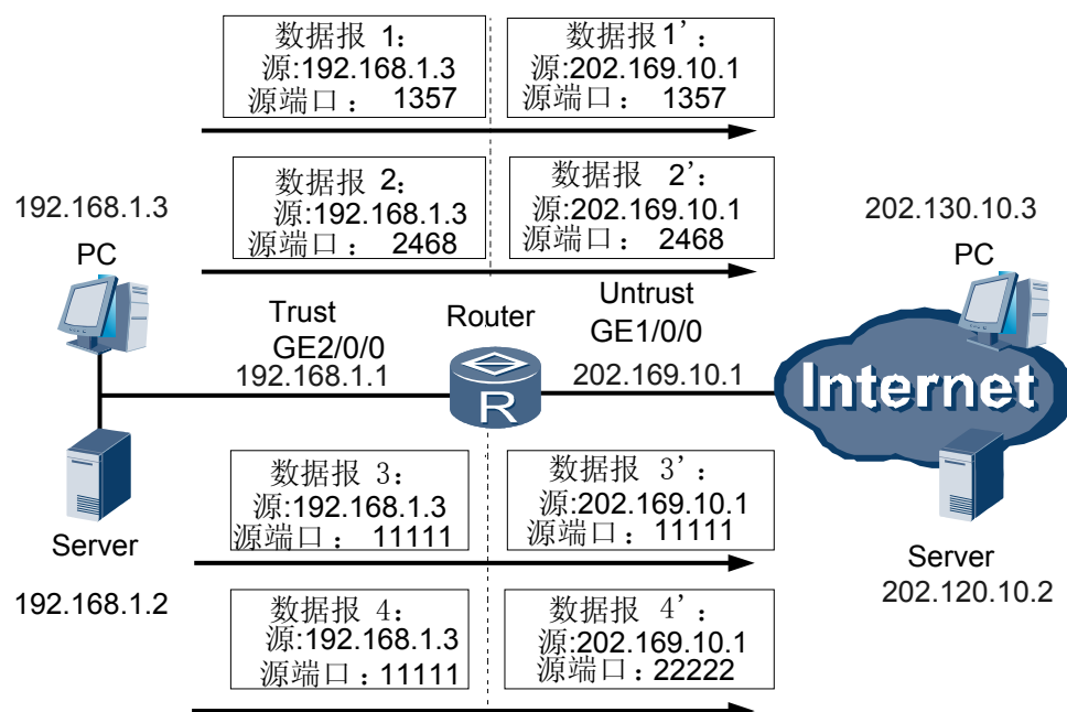
图 7-2 NAPT 示意图
