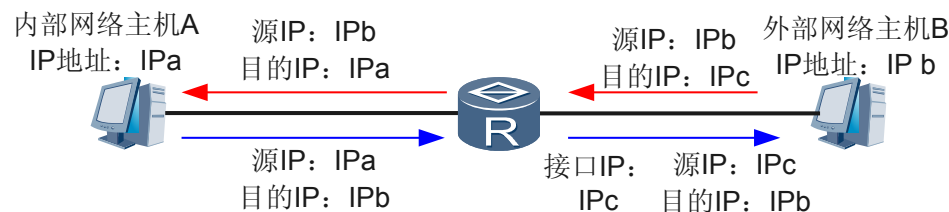
图 7-3 Easy IP 示意图
