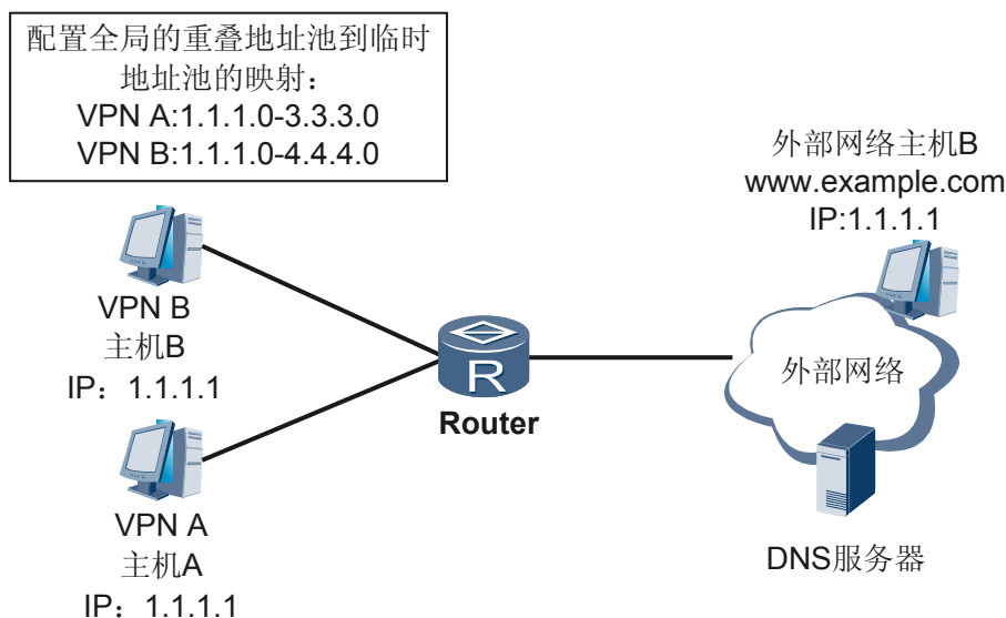
图 7-5 内网多 VPN 情况下的两次 NAT 示意图
