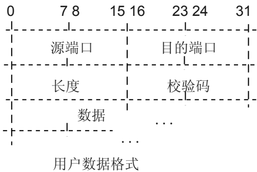
图 3-3 UDP 协议报文格式
