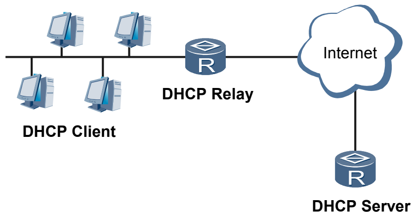
图 6-5 DHCP 中继的应用环境
