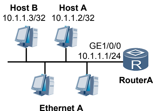
图 2-3 ARP-Ping IP 的实现过程
