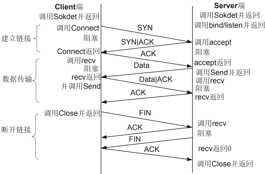
图 4-6 TCP6 连接建立和拆除过程示意图
