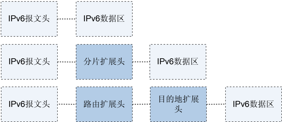
图 4-3 IPv6 扩展报文头
