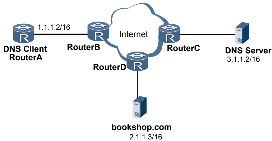
图 5-2 配置 DNS 客户端组网图
