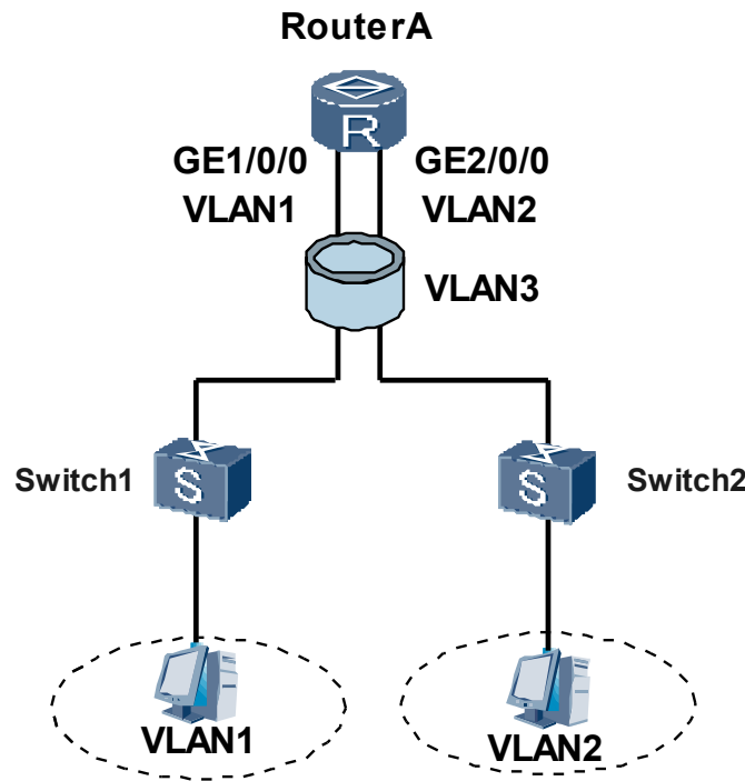
图 4-8 VLAN 间 ND 代理典型组网图
