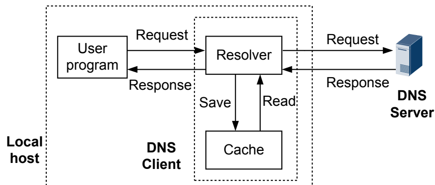
图 5-1 动态 DNS
